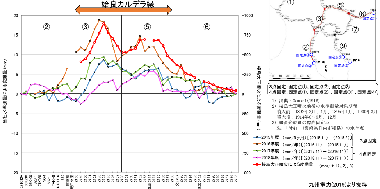
水準測量による垂直変化量の比較【基線②-③-⑤-⑥】
