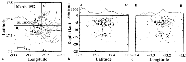
3月1日～29日の震源( M_c > 1.8 ) 分布
