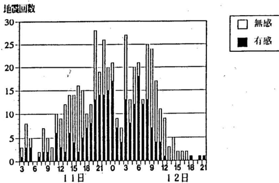
第1図 大正3年の桜島大噴火の前兆地震の推移(大森のデータに基づく) 1月11日から12日にかけての地震回数 (宇平, 1994; Omori(1920)のデータによる)
