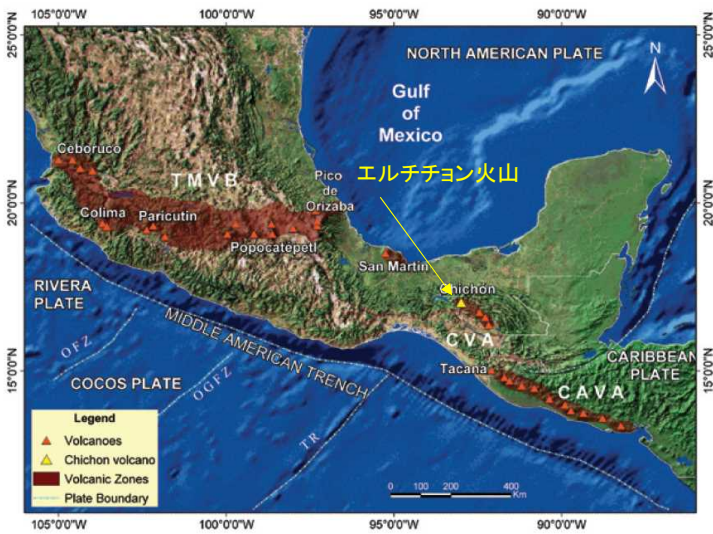
エルチヨン火山の位置 (Limon-Hernandez and Macias, 2009)
