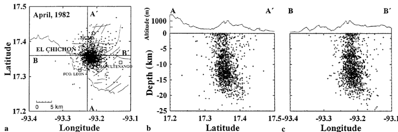
4月4日～27日の震源( M_c > 1.0 ) 分布
