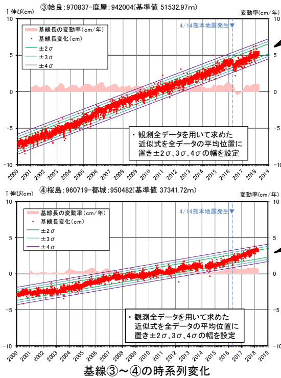
基線③~④の時系列変化
