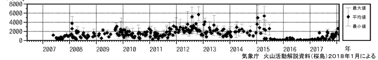
火山ガス(二酸化硫黄)の放出量
