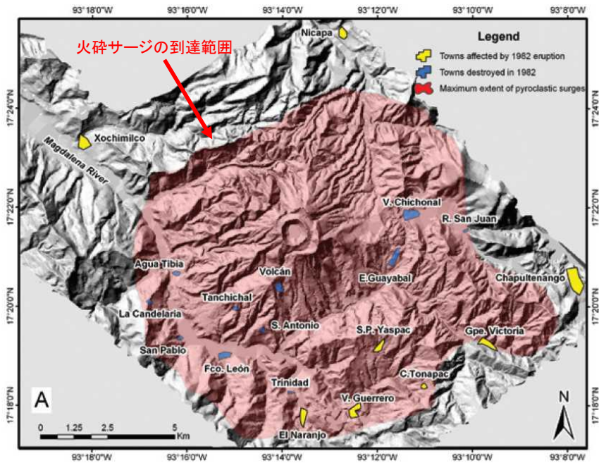
1982年4月4日主噴火の火砕流及びサージにより完全または部分的に消滅した町。B及びCは引用を省略。(Limon-Hernandez and Macias, 2009)
