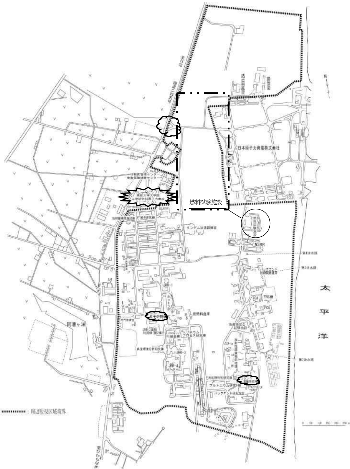
図4-1 国立研究開発法人日本原子力研究開発機構原子力科学研究所配置図
