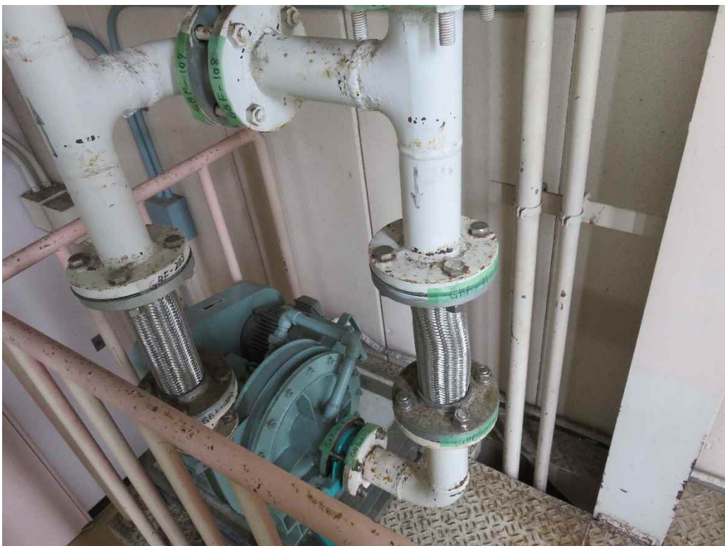
写真-2 送排風機
