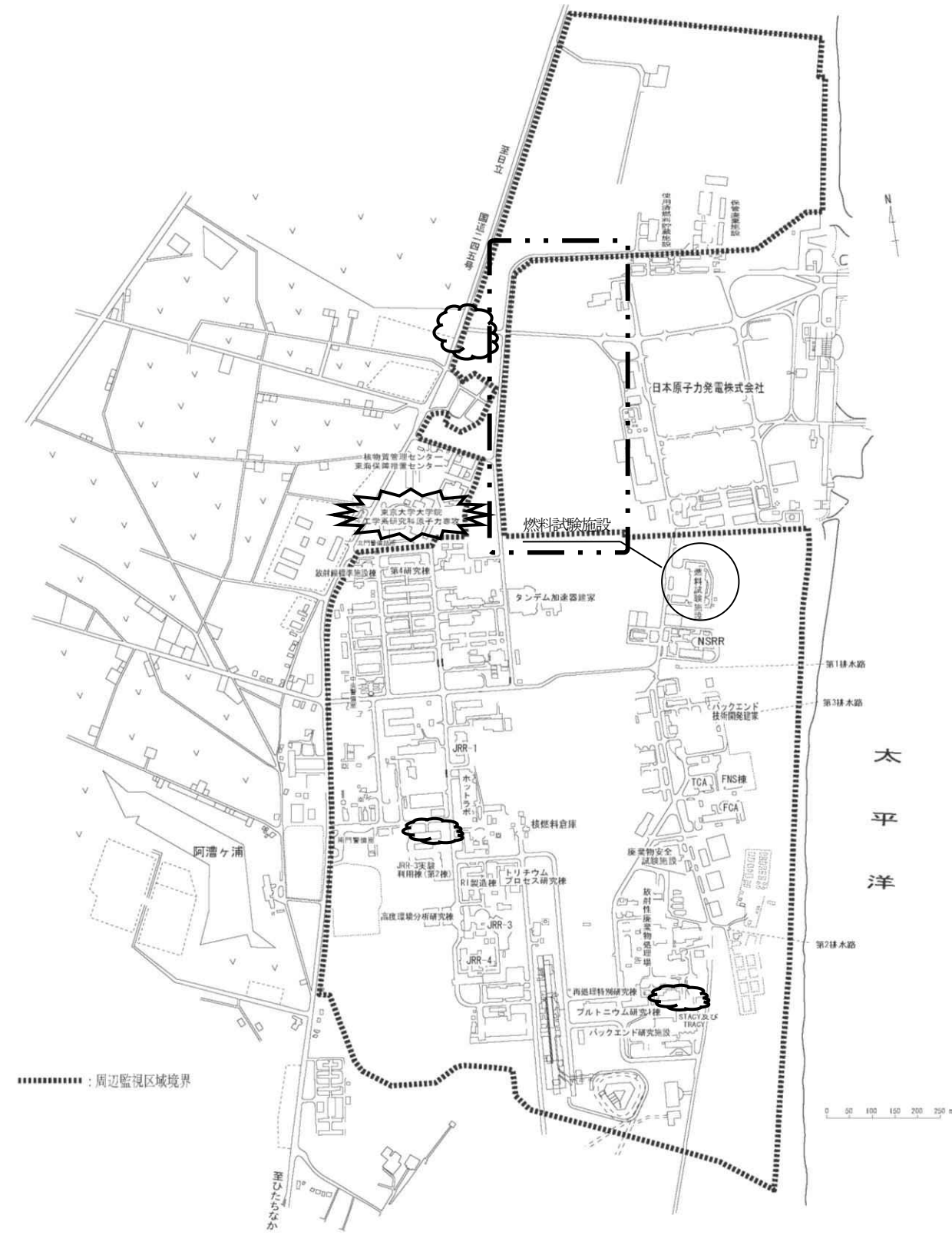
図4-1 国立研究開発法人日本原子力研究開発機構原子力科学研究所配置図
