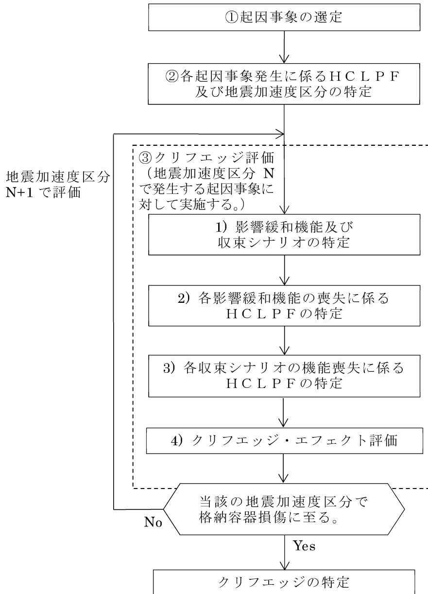
第 3.1.4.2.1.3 図 クリフエッジの特定に係るフロー図 (地震：格納容器損傷)
