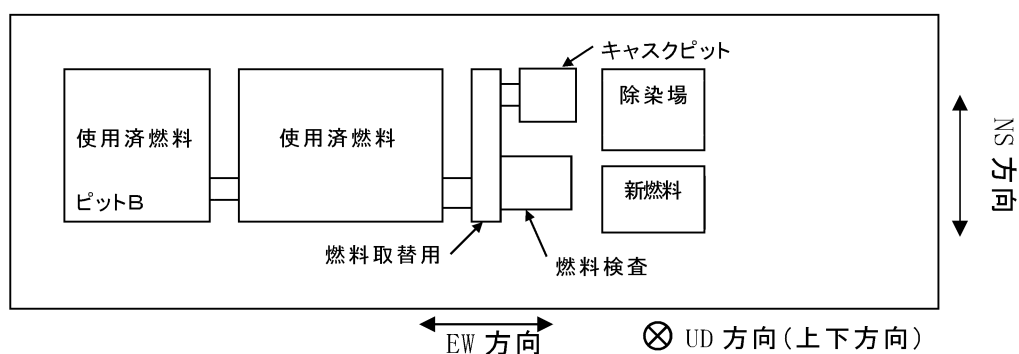
第 3.1.4.2.1.6 図 使用済燃料ピット周辺の概要図
