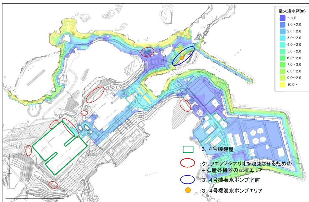
第 3.1.4.2.2.8 図 最大浸水深分布 (3, 4号機海水ポンプ室前潮位 : E.L.+11.4m)
