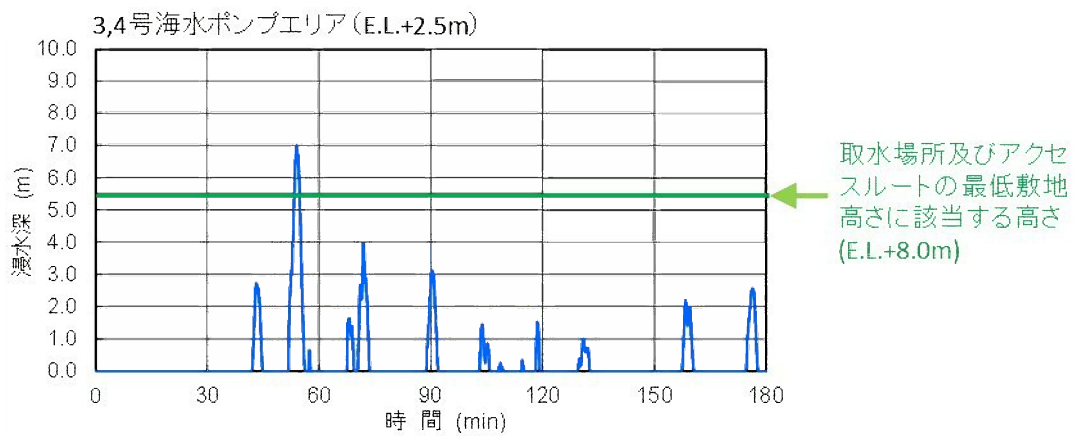
第 3.1.4.2.2.14 図 3 , 4 号機海水ポンプエリア (E.L.+2.5m) の津波水位変化
