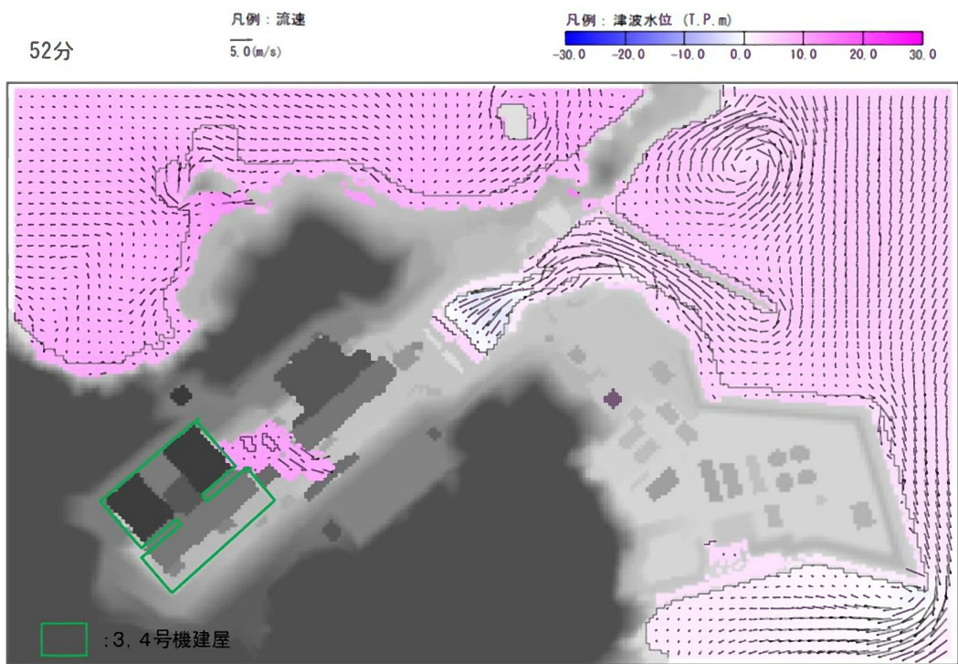
第 3.1.4.2.2.13 図 流速ベクトル分布 ( 3 , 4 号機海水ポンプ室前潮位 : E.L.+9.9m)
