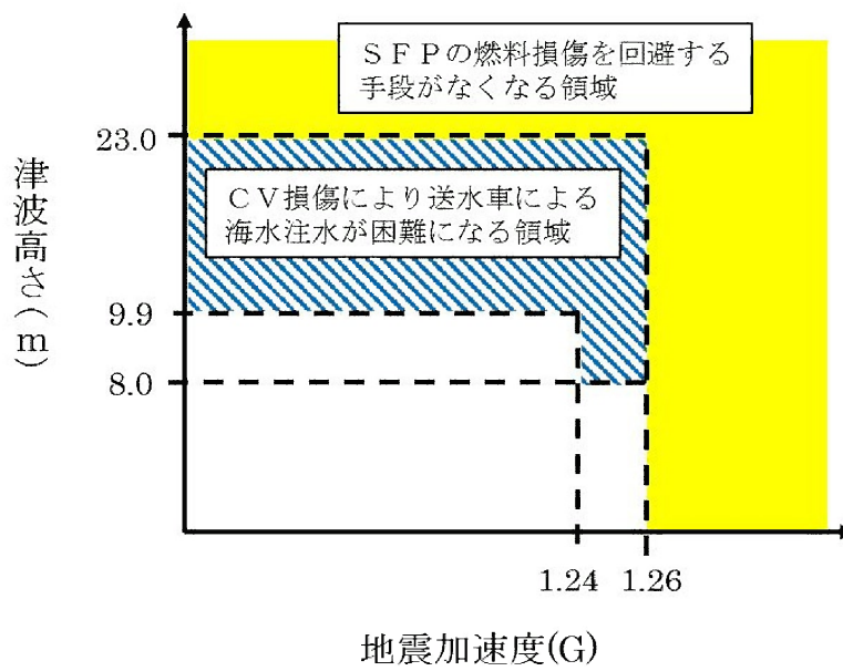
第 3.1.4.2.3.9 図 遡上を考慮した地震と津波の重畳に関するクリフエッジ評価結果（SFP 燃料損傷）
