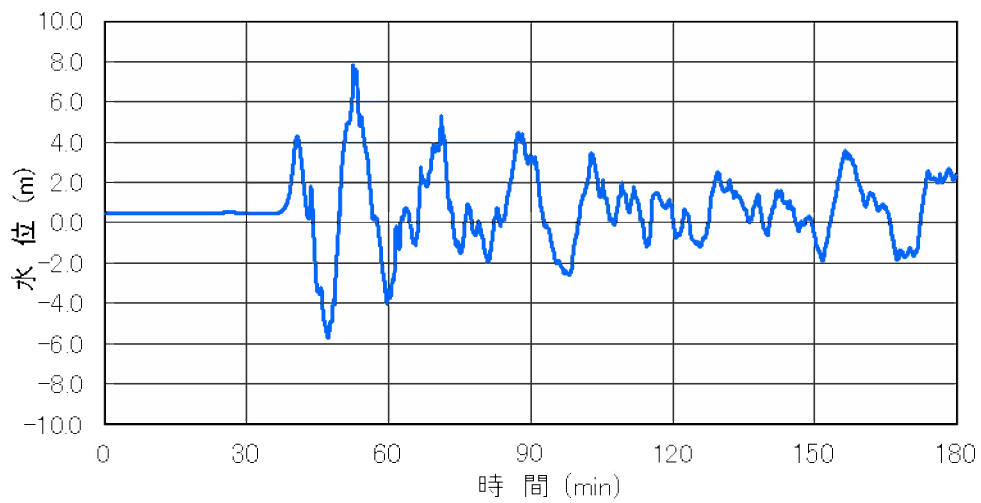
第 3.1.4.2.2.6 図 遡上解析で想定する入力津波の時刻歴波形 (鋸崎から約 1km 離れた海域 (水深 40m 地点)) (3, 4 号機海水ポンプ室前潮位 : E.L.11.4m) (初期潮位 : E.L. + 0.49m)
