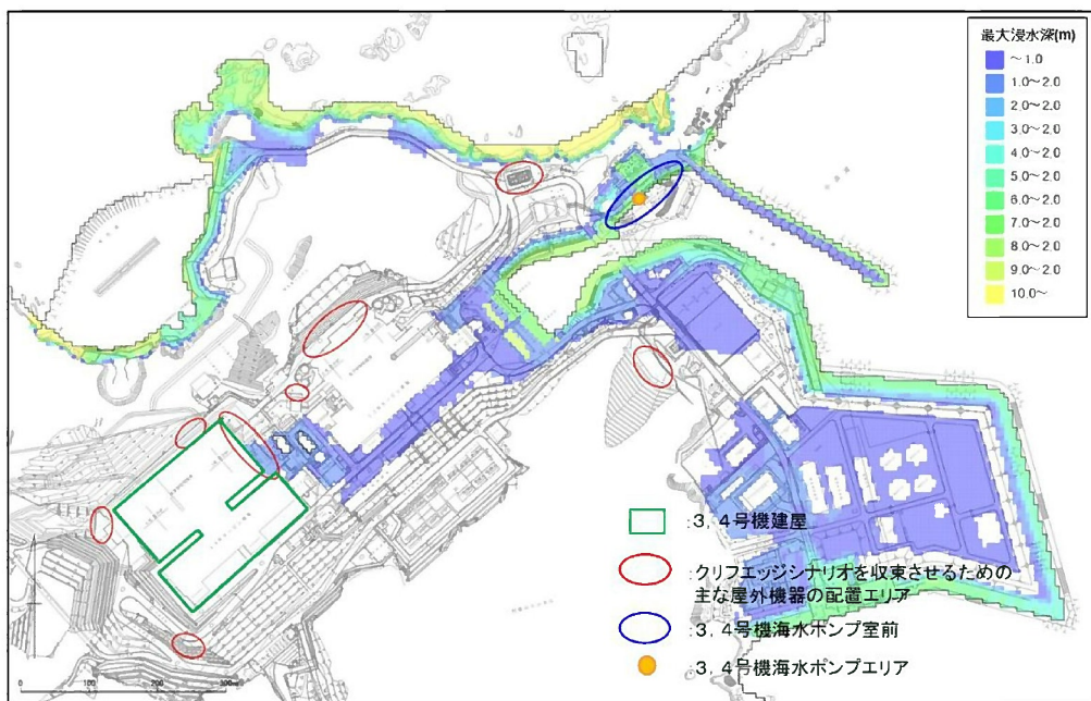
第 3.1.4.2.2.12 図 最大浸水深分布 (3, 4号機海水ポンプ室前潮位 : E.L.+9.9m)
