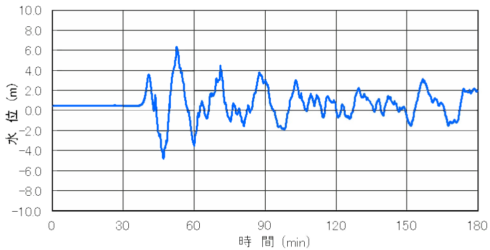
第 3.1.4.2.2.10 図 遡上解析で想定する入力津波の時刻歴波形 ( 鋸崎から約 1km 離れた海域 (水深 40m 地点) ) ( 3 , 4 号機海水ポンプ室前潮位 : E.L.+9.9m ) ( 初期潮位 : E.L.+0.49m )
