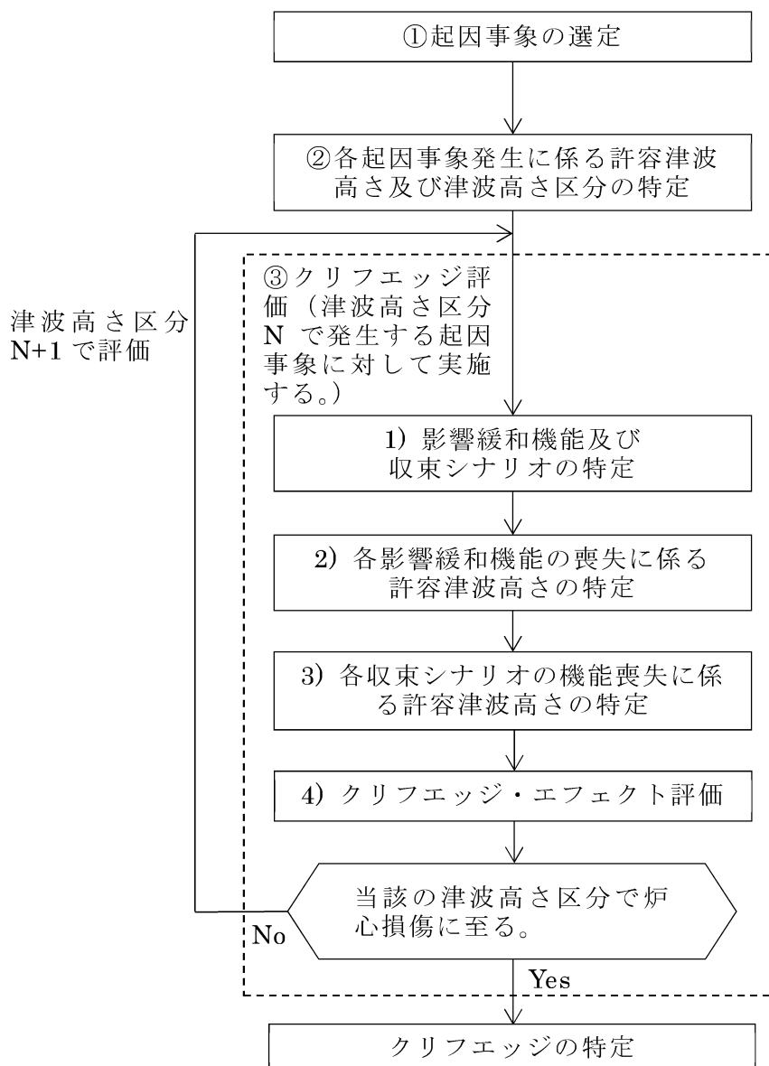
第 3.1.4.2.2.2 図 クリフエッジの特定に係るフロー図
