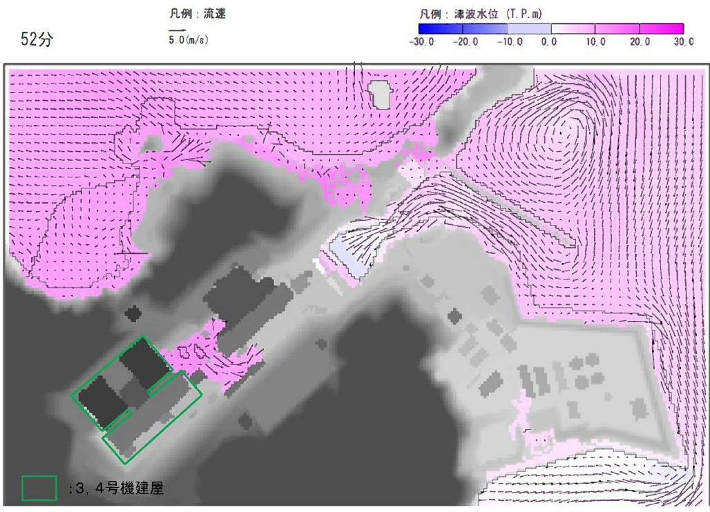
第 3.1.4.2.2.9 図 流速ベクトル分布 ( 3 , 4 号機海水ポンプ室前潮位 : E.L.+11.4m )
