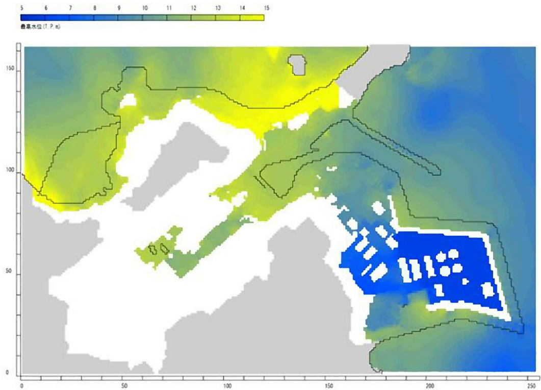
第 3.1.4.2.2.7 図 最高水位分布 (3, 4号機海水ポンプ室前潮位 : E.L.+11.4m)
