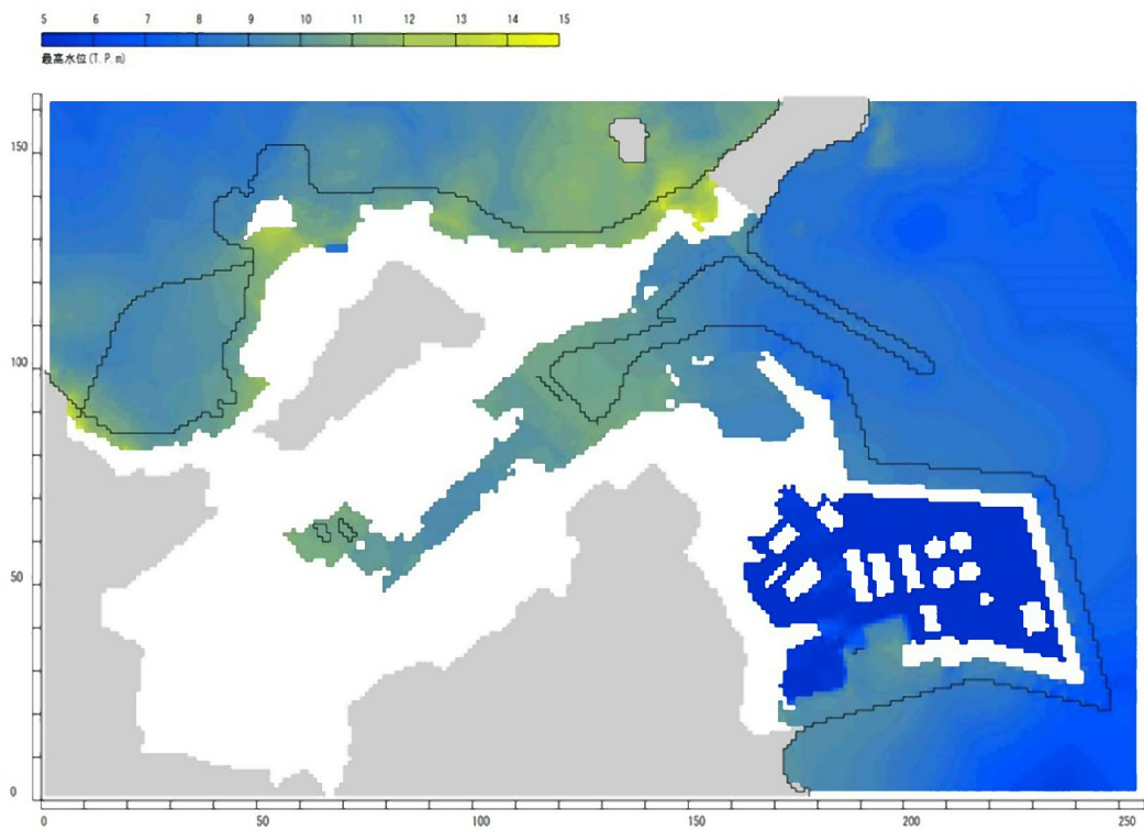
第 3.1.4.2.2.11 図 最高水位分布 (3, 4号機海水ポンプ室前潮位 : E.L.+9.9m)
