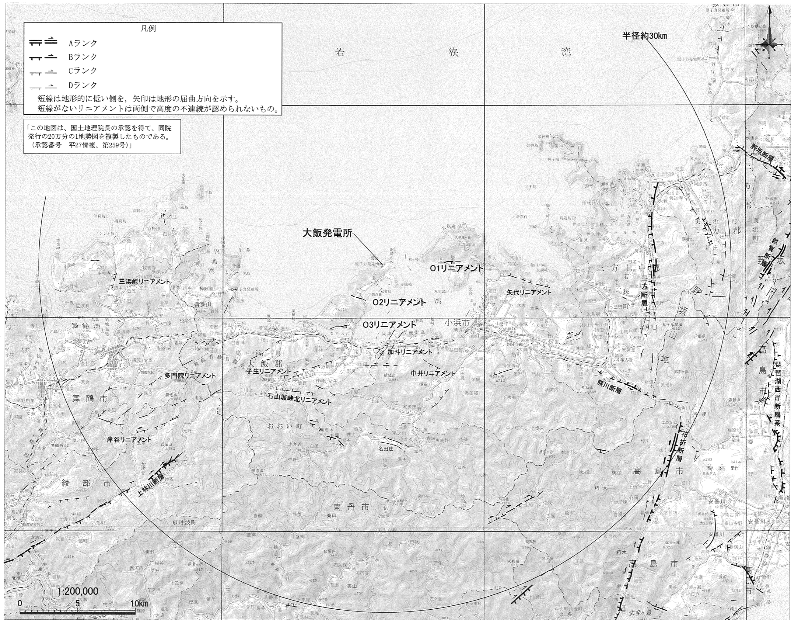
第1.2.3.1.6図 敷地周辺陸域の変動地形・リニアメント分布図
