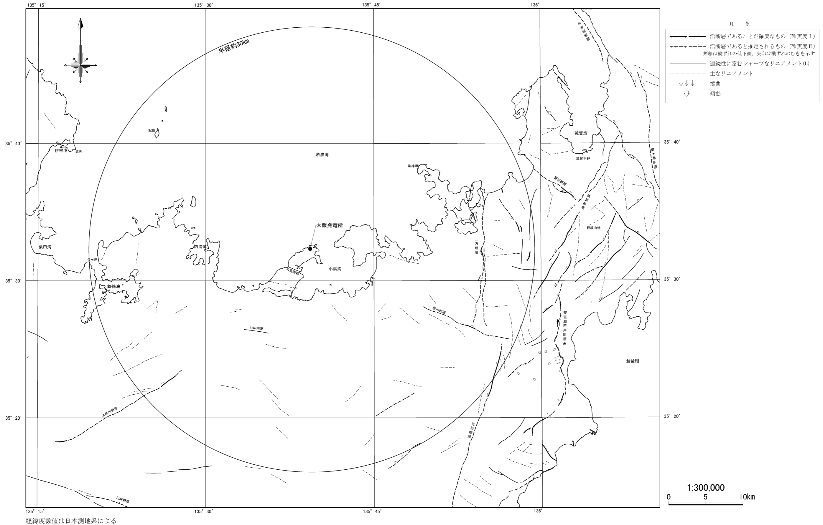
第1.2.3.1.4図 敷地周辺陸域の活断層分布図 「近畿の活断層」
