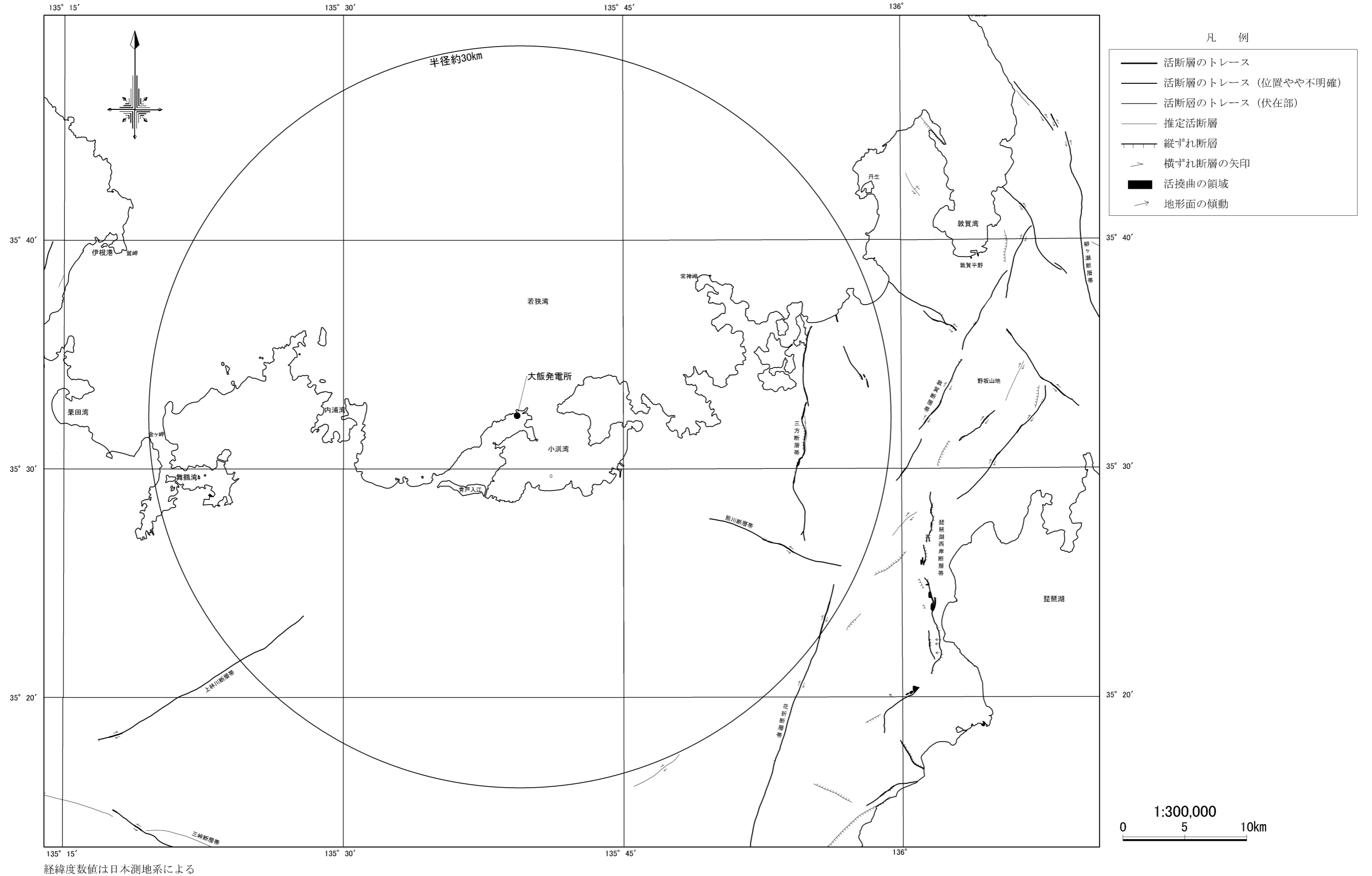
第1.2.3.1.5図 敷地周辺陸域の活断層分布図 「活断層詳細デジタルマップ」
