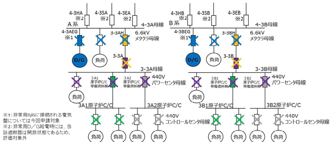
第2-2図 アーク放電発生箇所とアーク放電を遮断する遮断器
