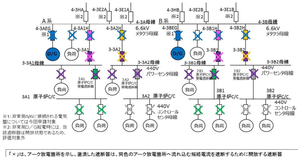
第2-2図 アーク放電発生箇所とアーク放電を遮断する遮断器 (非常用ディーゼル発電機給電時)
