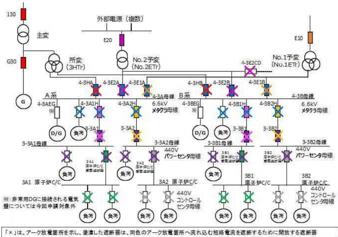
第2-1図 アーク放電発生箇所とアーク放電を遮断する遮断器 (非常用ディーゼル発電機給電時以外)
