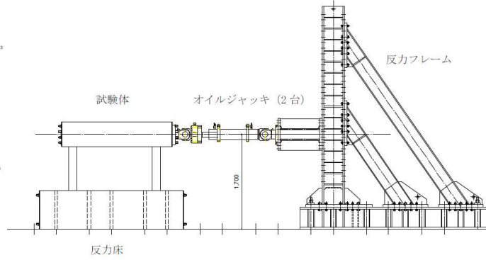
加力装置
