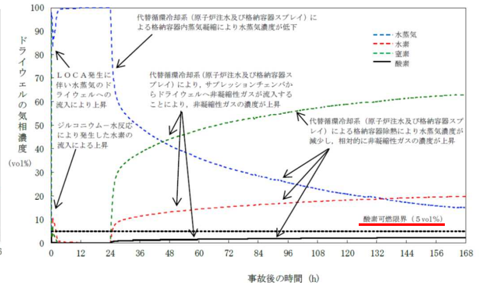
ドライウエルの気相濃度の推移(ウェット条件)
