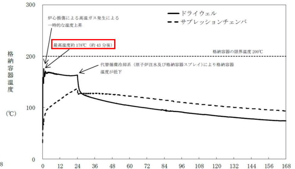
原子炉格納容器雰囲気温度の推移
