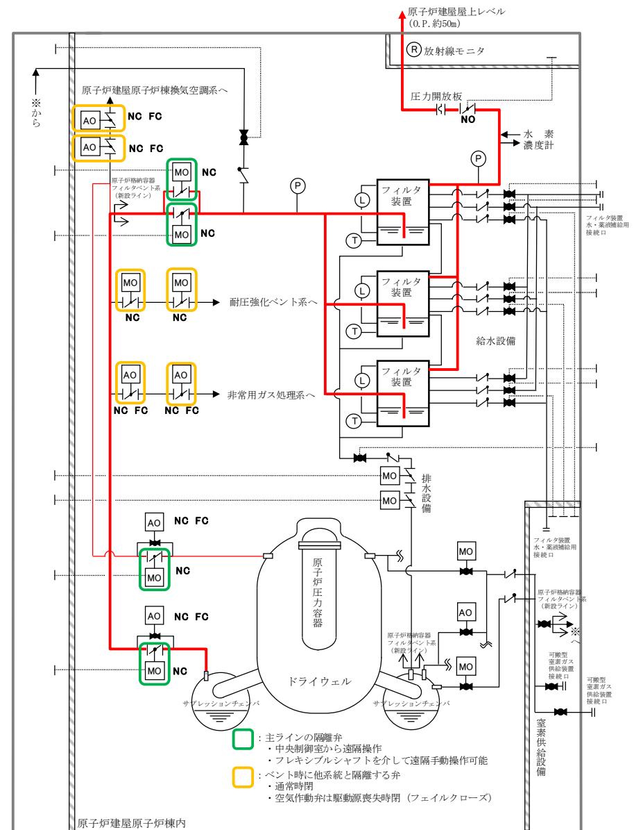
原子炉建屋
