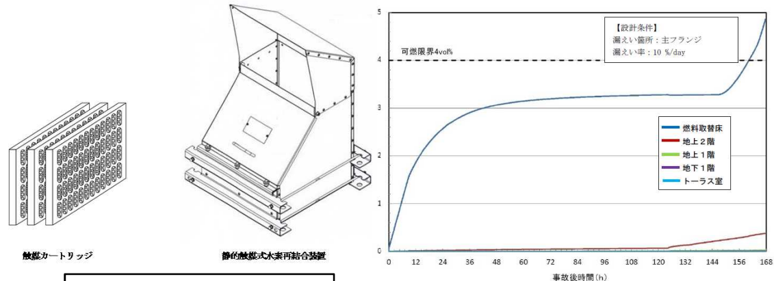
静的触媒式水素再結合器
