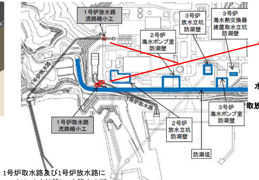
取放水路流路縮小工の概要図
