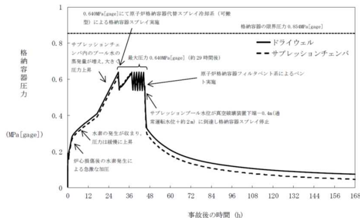
格納容器圧力の推移
