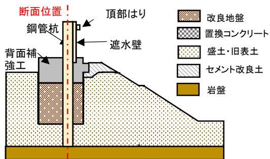
変更前の鋼管式鉛直壁(一般部)の構造概要
