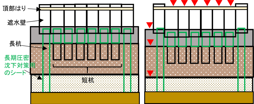
変更前の断面図(通常時)
