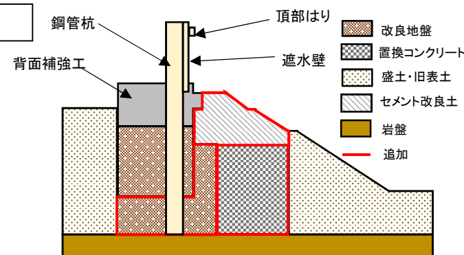
変更後の鋼管式鉛直壁(一般部)の構造概要
