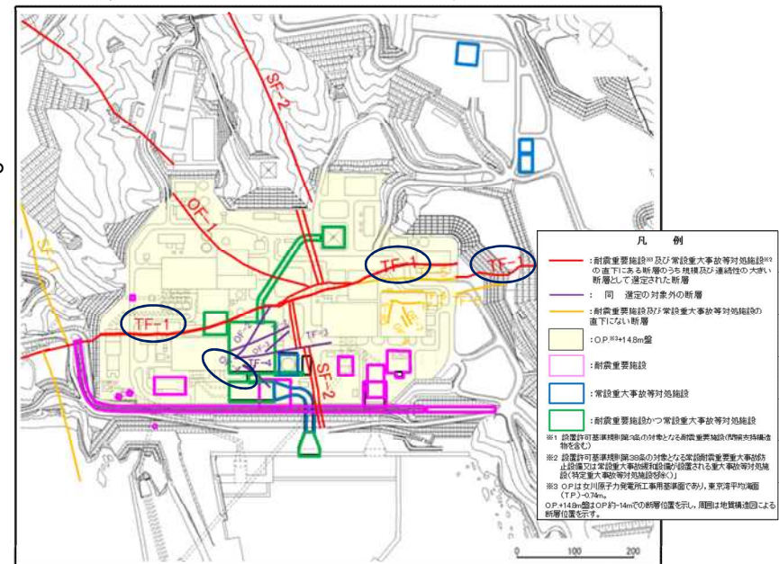
【敷地内の検討対象断層と耐震重要施設等の位置】
