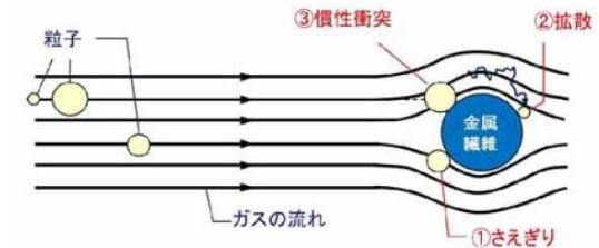
金属フィルタによる除去原理(イメージ)
