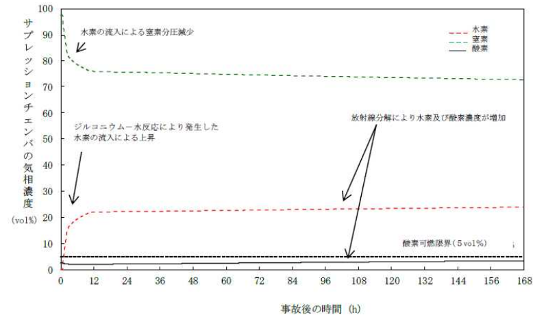
代替循環冷却系を使用した場合のサプレッションチェンバの気相濃度の推移(ドライ条件)
