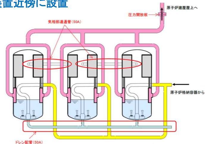
フィルタ装置周りの系等概要図
