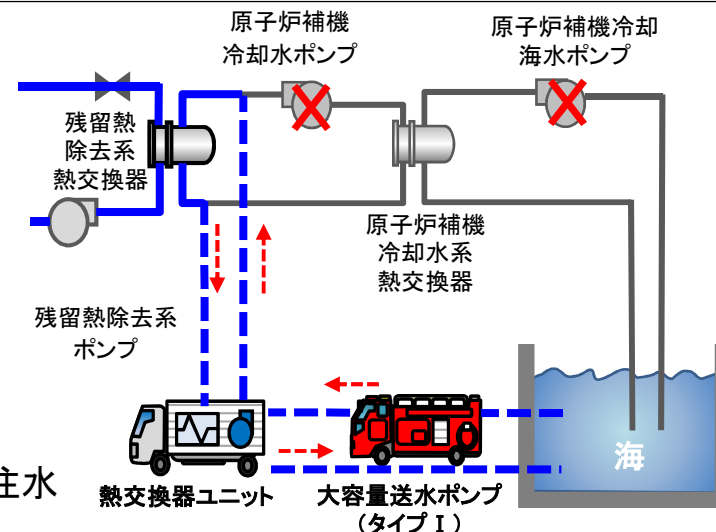
原子炉補機代替冷却水系
