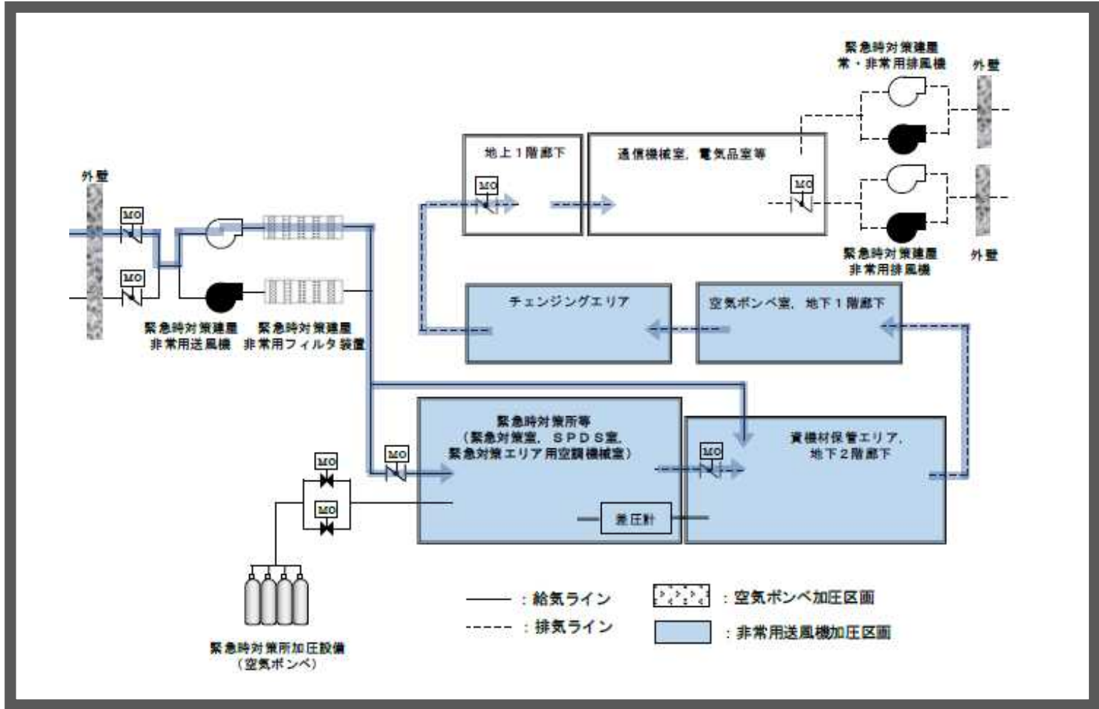
設備(換気空調系概要図)
