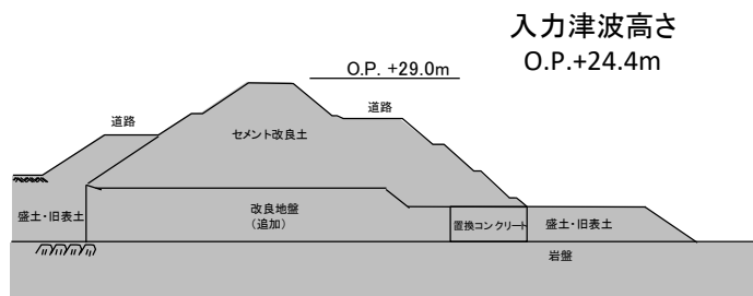
盛土堤防の概要図(断面図)
