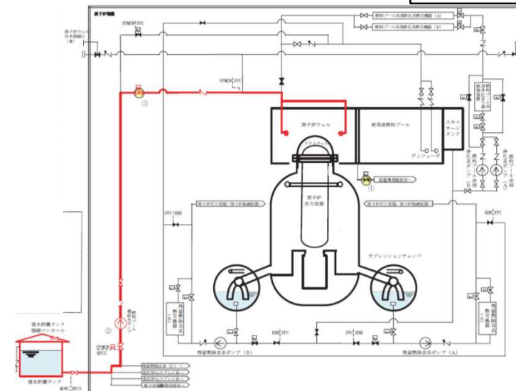
格納容器頂部注水系
