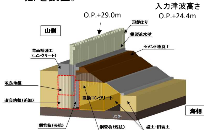
防潮堤(鋼管式鉛直壁)の概要図
