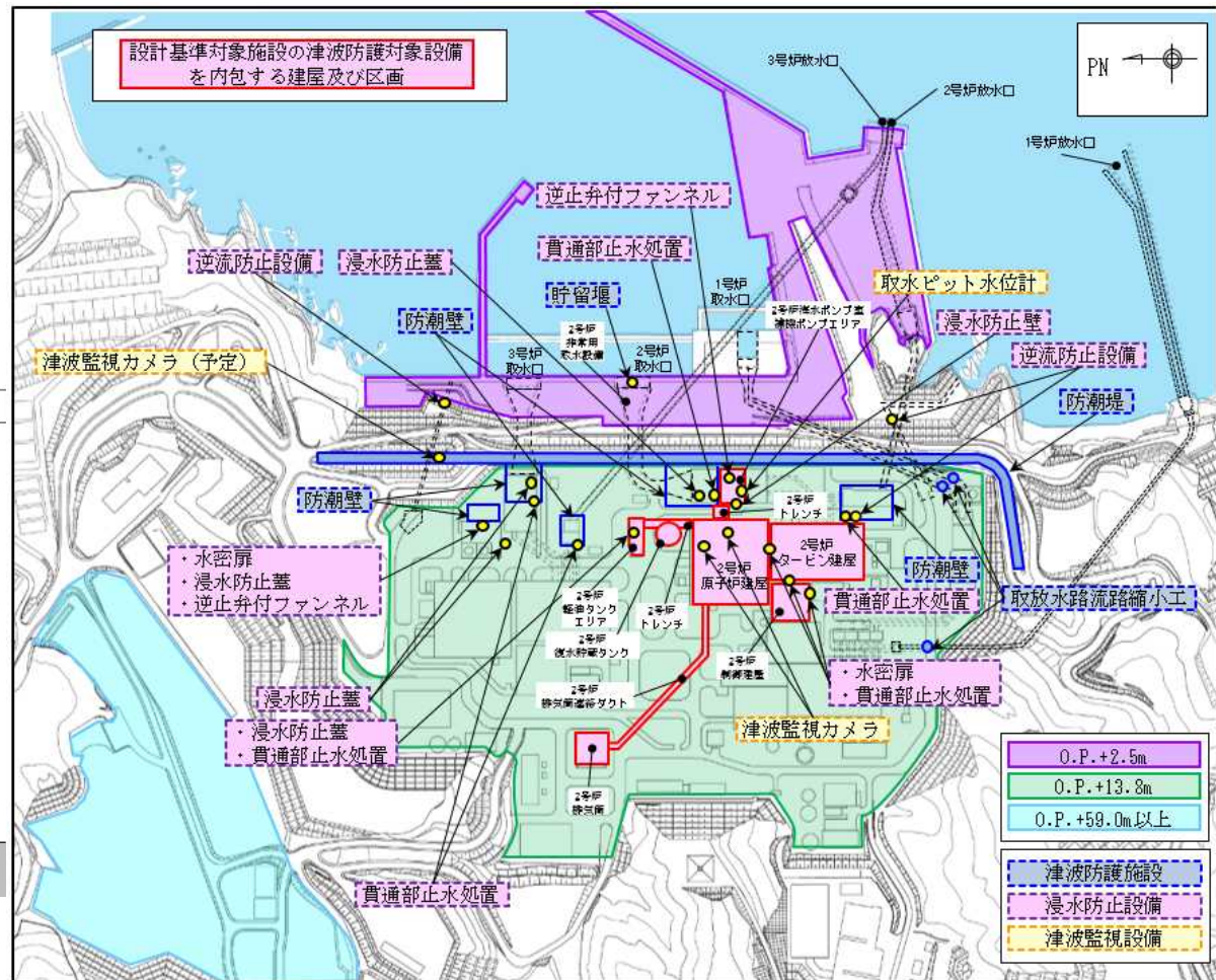
敷地の特性に応じた津波防護の概要
