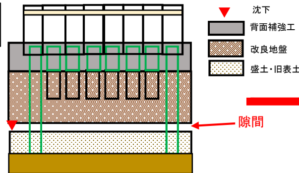
シートが機能しなかった場合の断面図(地震時)
