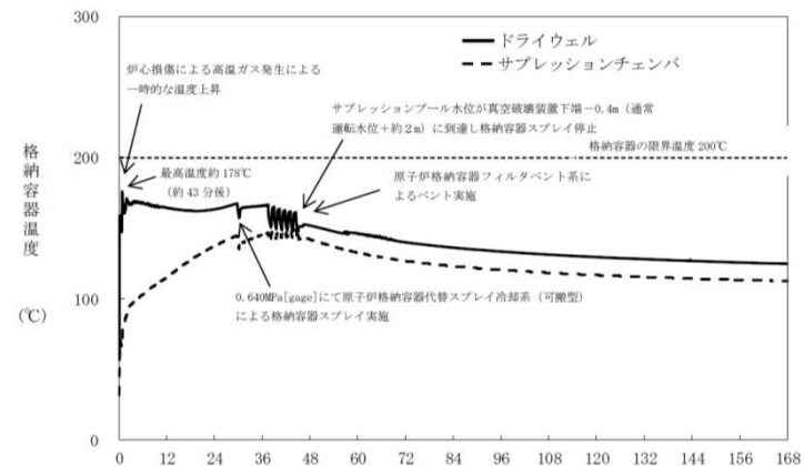
格納容器温度の推移
