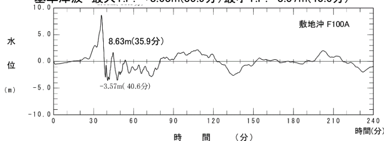
【基準津波定義位置における水位時刻歴波形※1】
