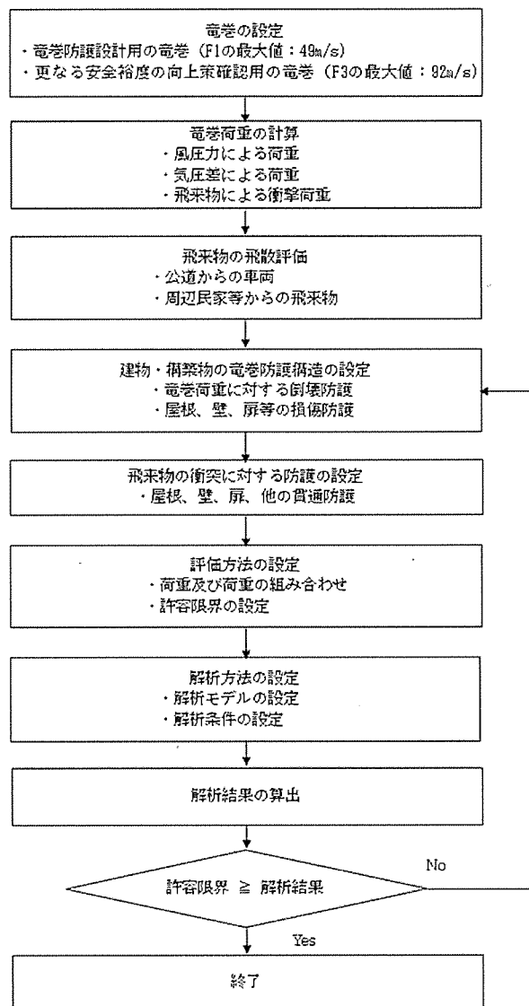
添設建 3-I.1 図 建物・構築物の竜巻防護設計フロー概要
