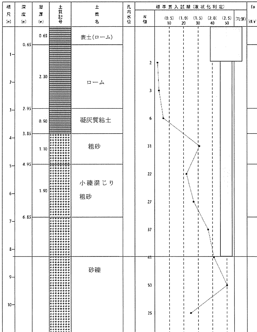
添説建 2-Ⅱ. 1.9-2 図 ボーリング柱状図 (①地点)
