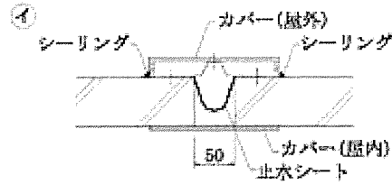
添説建2付2-2図 エキスパンションジョイント構造例の概要
