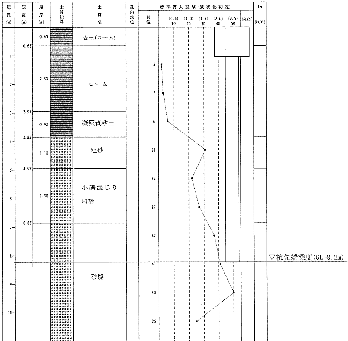
添説建 2-III. 1.9-2 図 ボーリング柱状図 (①地点)
