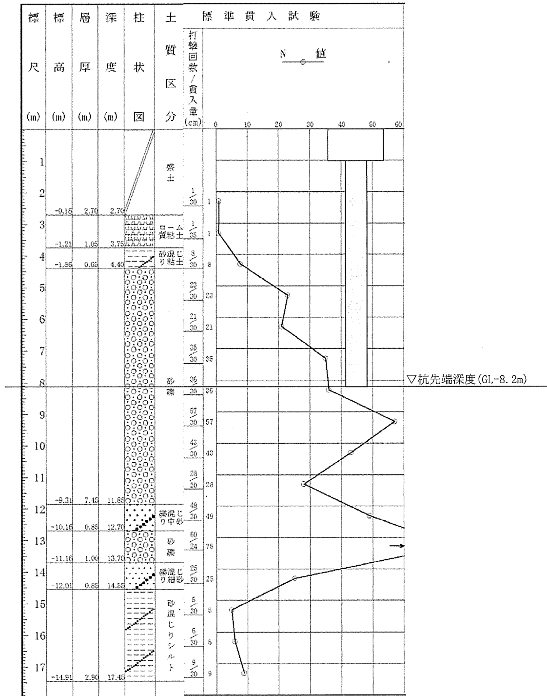
添説建 2-III. 1. 9-3 図 ボーリング柱状図 (②地点)
