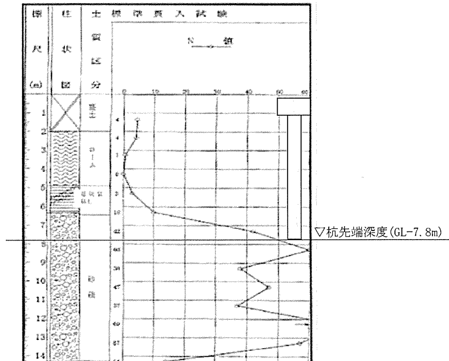
添説建 2-V.1.9-3 図 ボーリング柱状図 (②地点)
