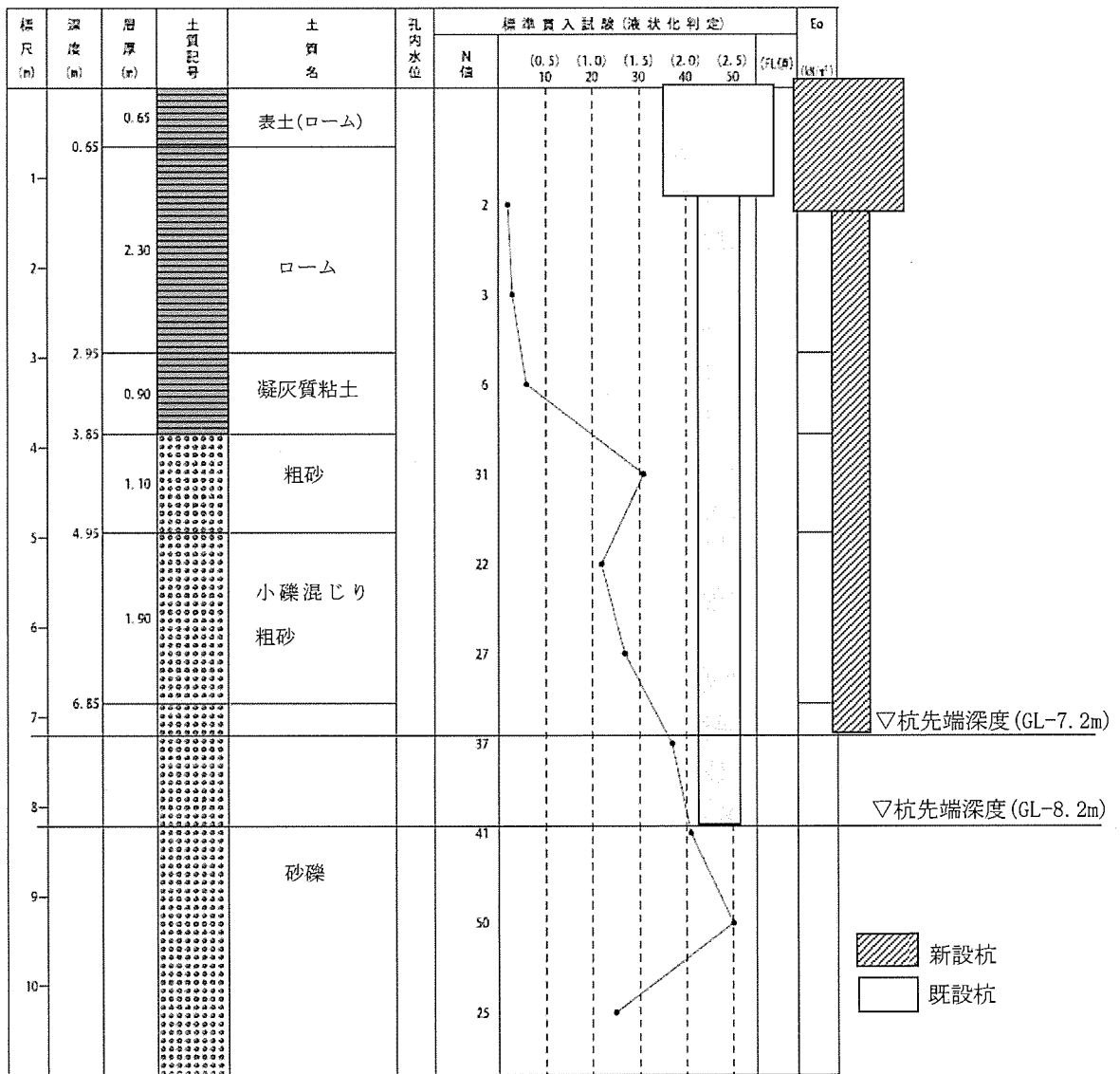
添説建 2-IV. 1.9-2 図 ボーリング柱状図 (①地点)
