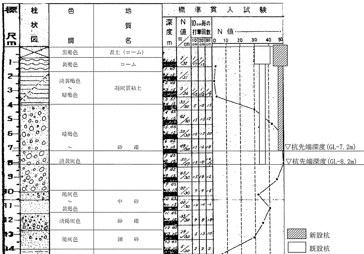
添説建 2-IV. 1.9-3 図 ボーリング柱状図 (②地点)
