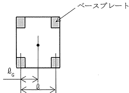
A-A断面図
