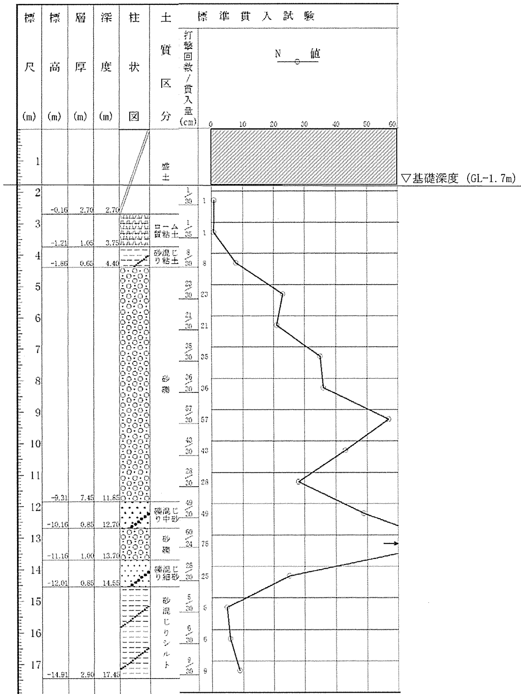
添説建 2-VIII. 1.8-3 図 ボーリング柱状図 (②地点)
