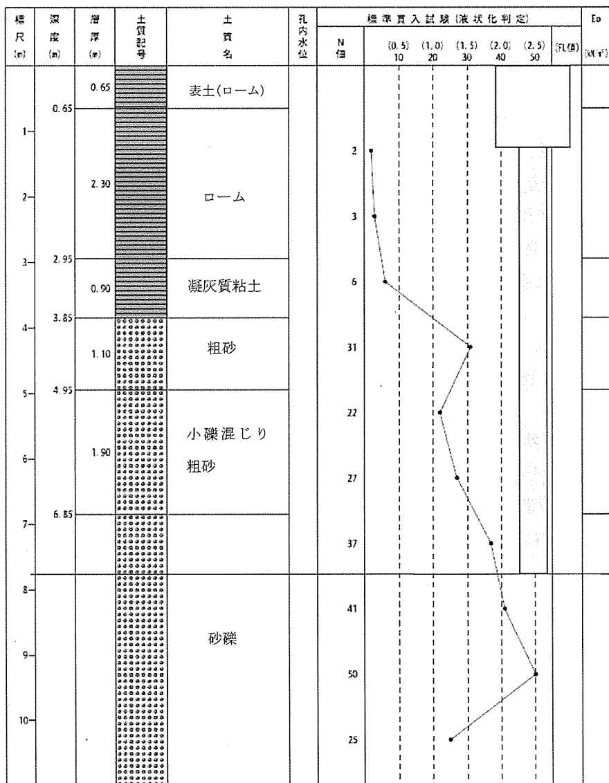
添説建 2-V.1.9-2 図 ボーリング柱状図 (①地点)
