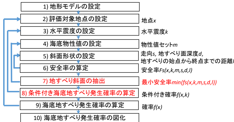
図2 海底地すべりの発生確率の算定手順（変更前）
