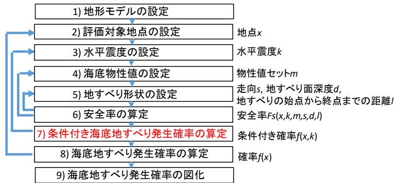
図1 海底地すべりの発生確率の算定手順（変更後）
