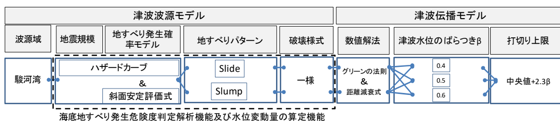
図3 海底地すべり起因津波のロジックツリー（案）
