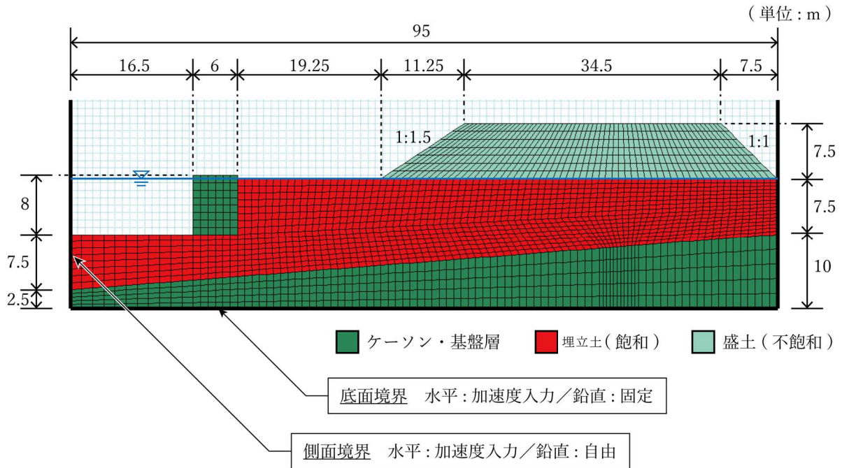
図-1 密な地盤及び緩い地盤の解析モデル（メッシュ分割のイメージ）
