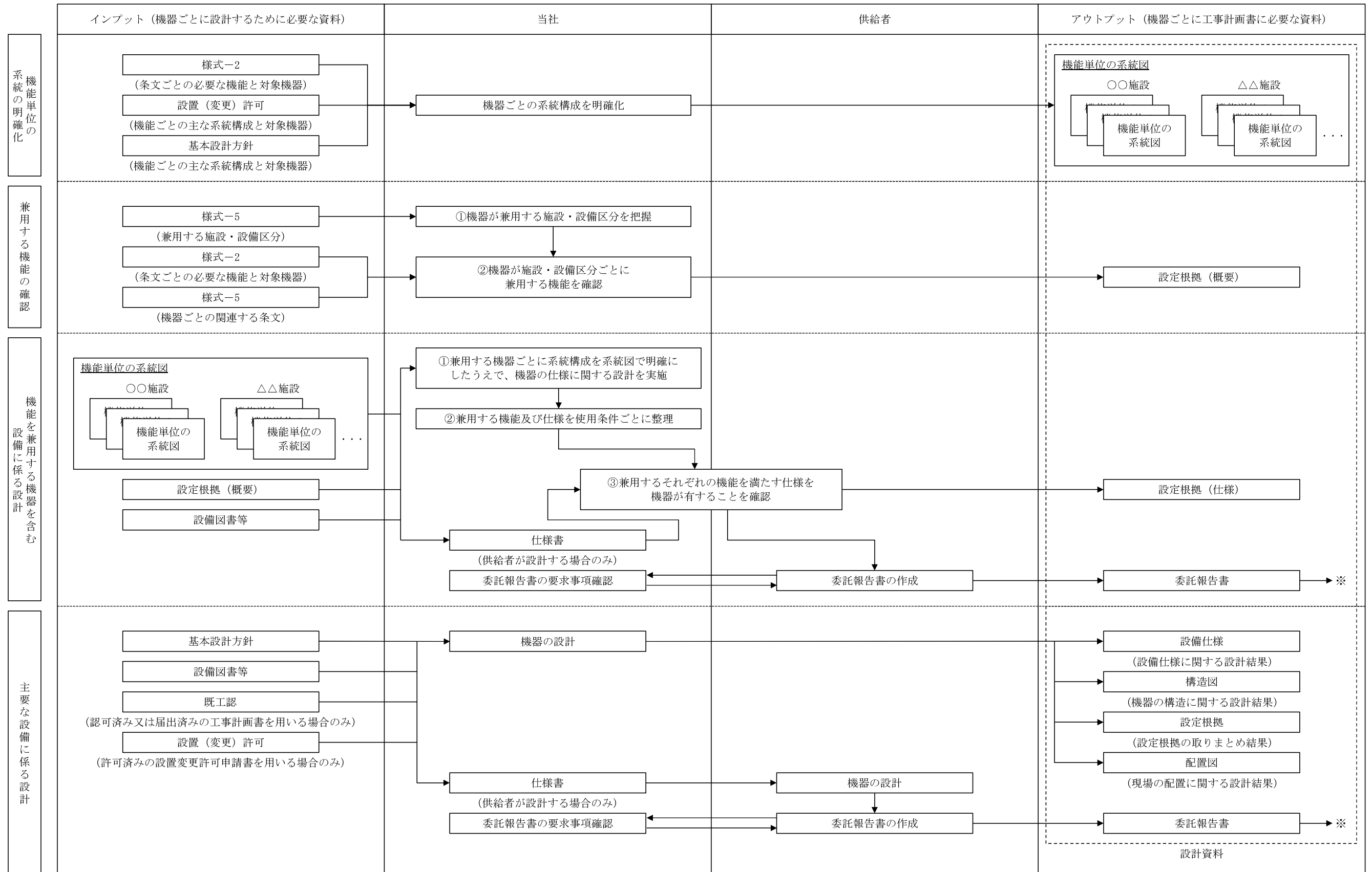
第5図 主要な設備の設計
