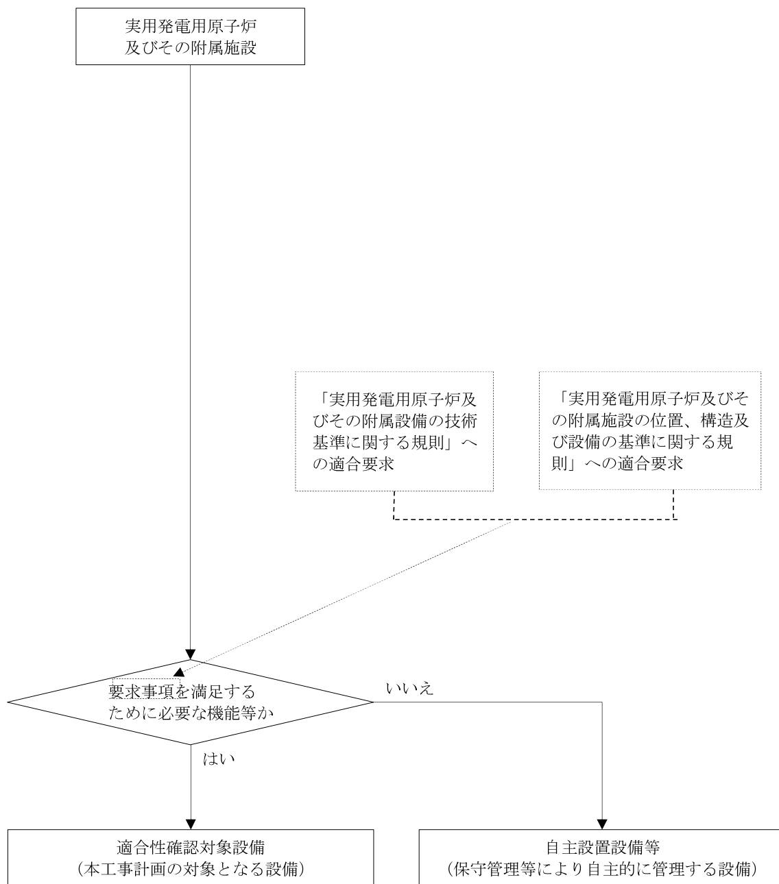
第4図 適合性確認対象設備の抽出について
