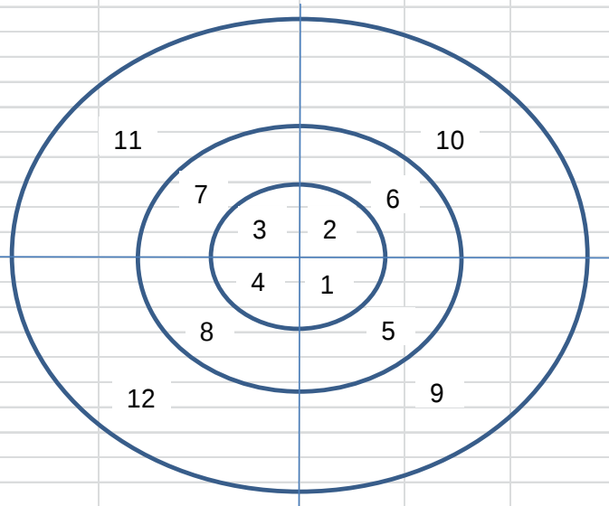
図3 CCTF 実験解析の炉心領域セル分割（直交座標系）
