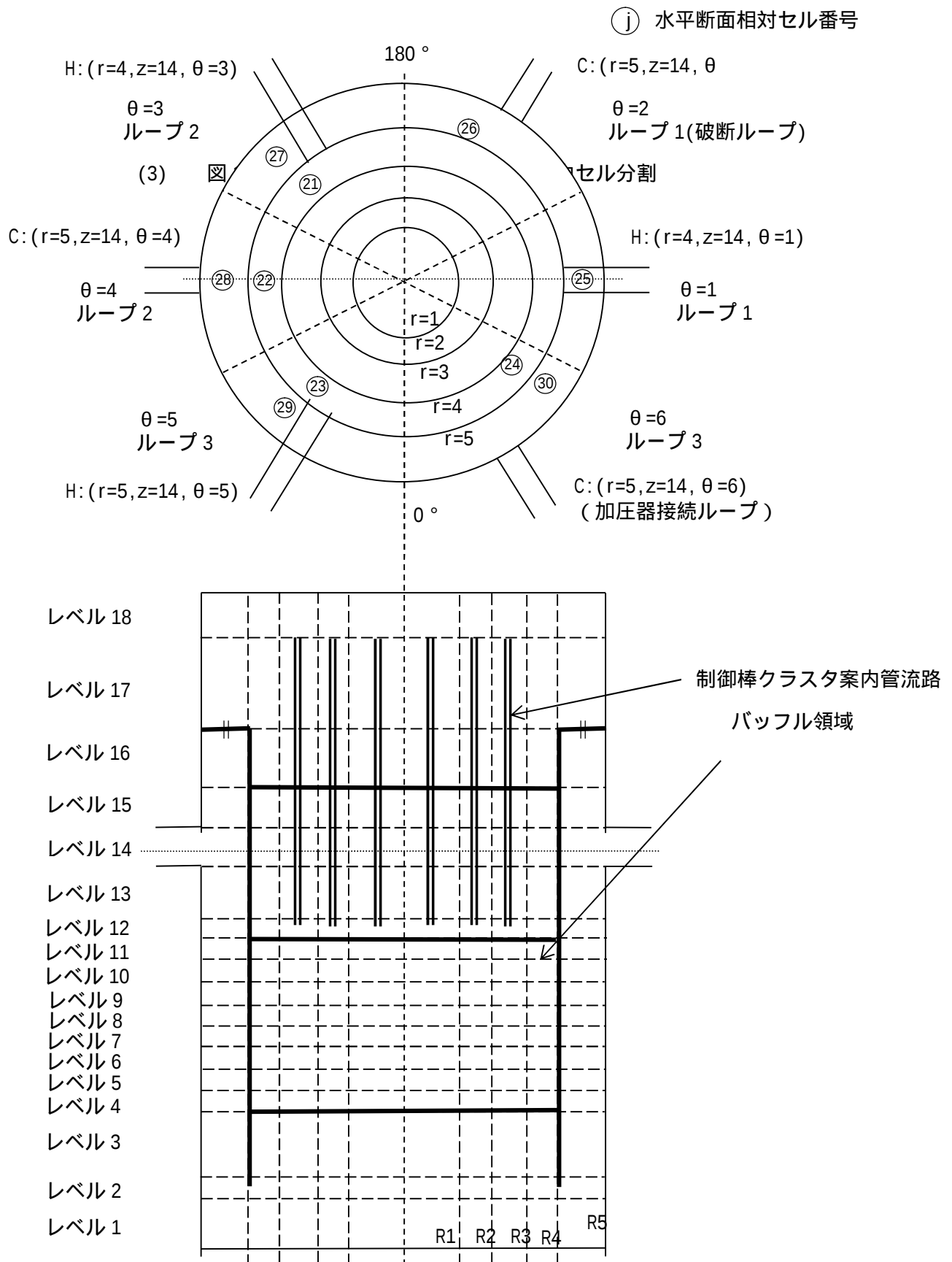
図5 PWR 3 ループプラントの原子炉容器内の炉心領域を除くセル分割
