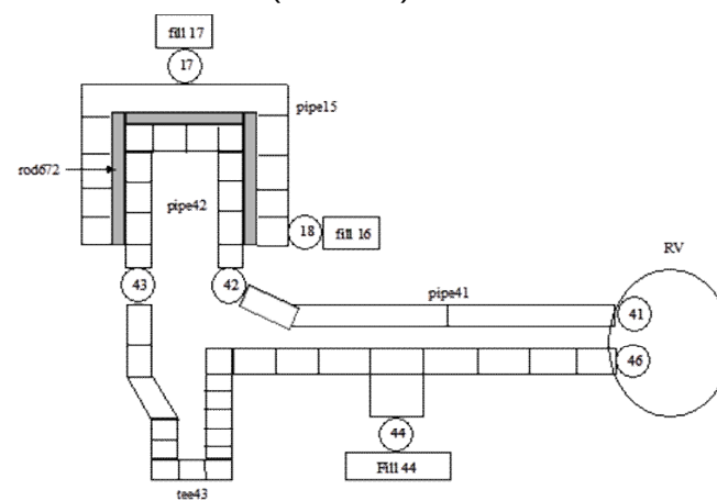
健全ループ(ループ 4)
