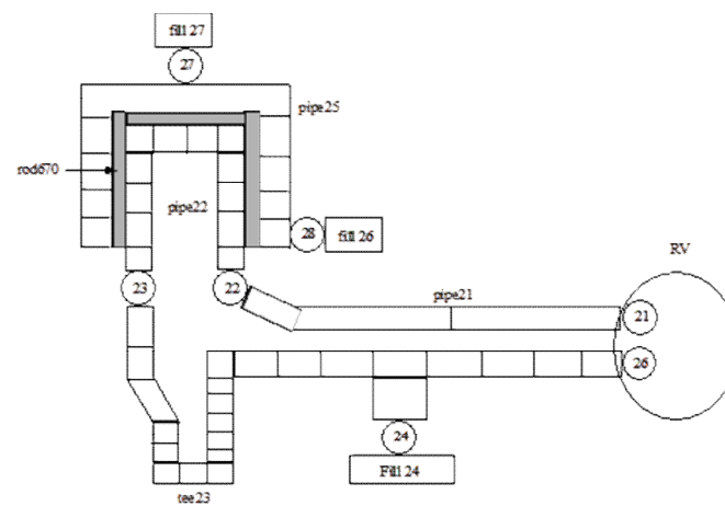
健全ループ(ループ 2)
