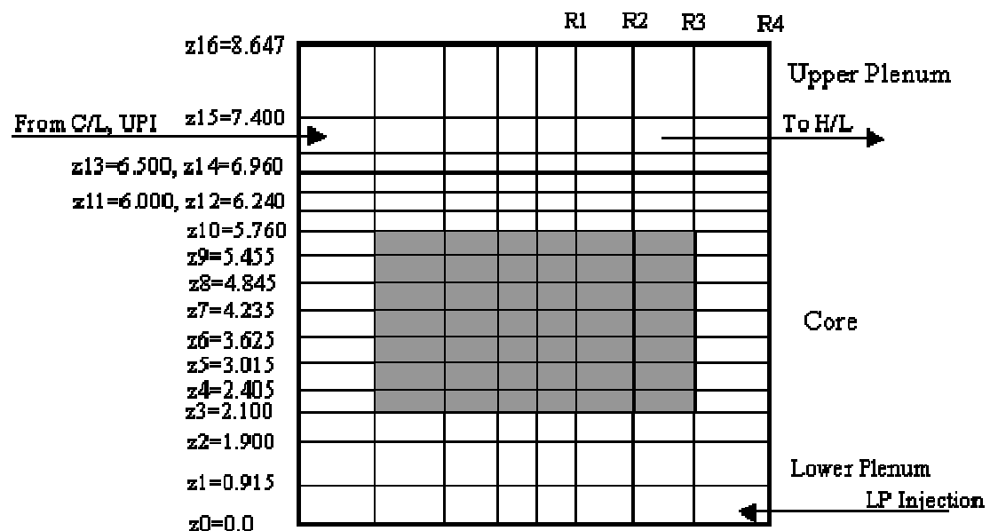
図 2 CCTF 実験解析の原子炉容器内セル分割
