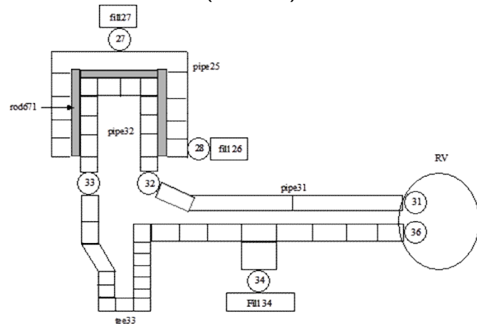
健全ループ(ループ 3)
