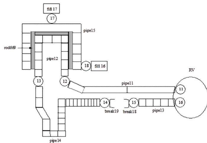
破断ループ(ループ 1)
