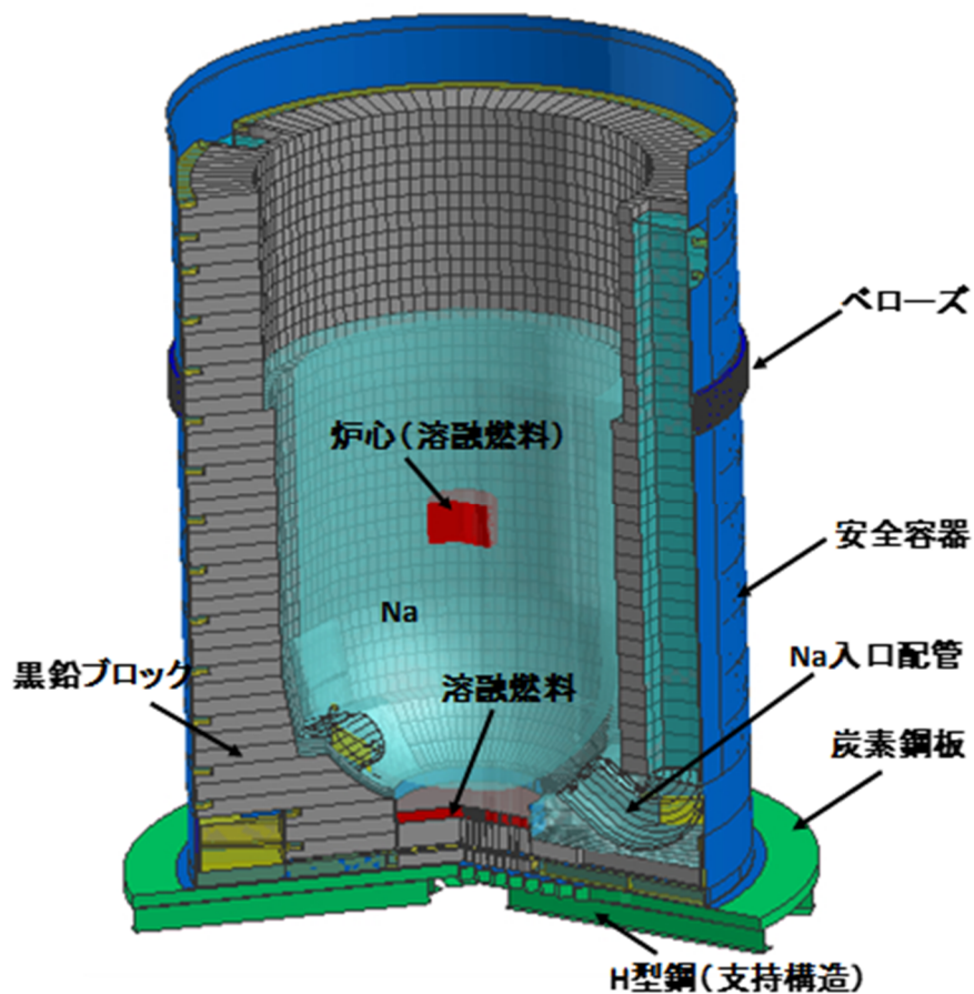
図 1 原子炉容器外容器の解析モデル (平成 30 年度モデル): 参考用
