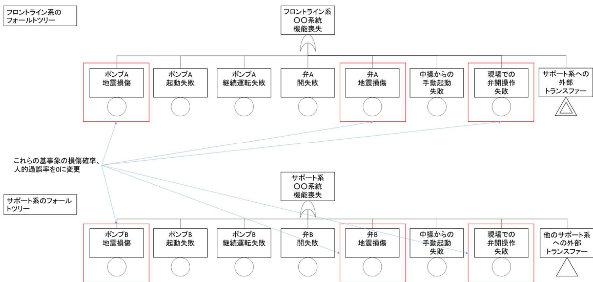
図 5 ランダム故障のみによる系統機能喪失確率の計算のイメージ
