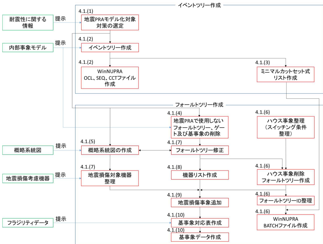
図 1 プラント A のモデル作成フロー
