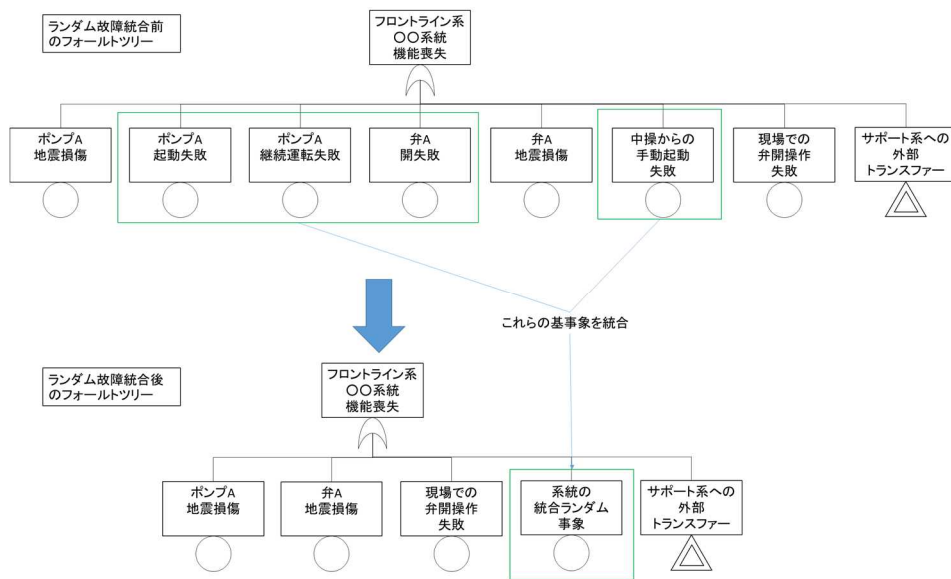
図 6 ランダム故障の統合のイメージ
