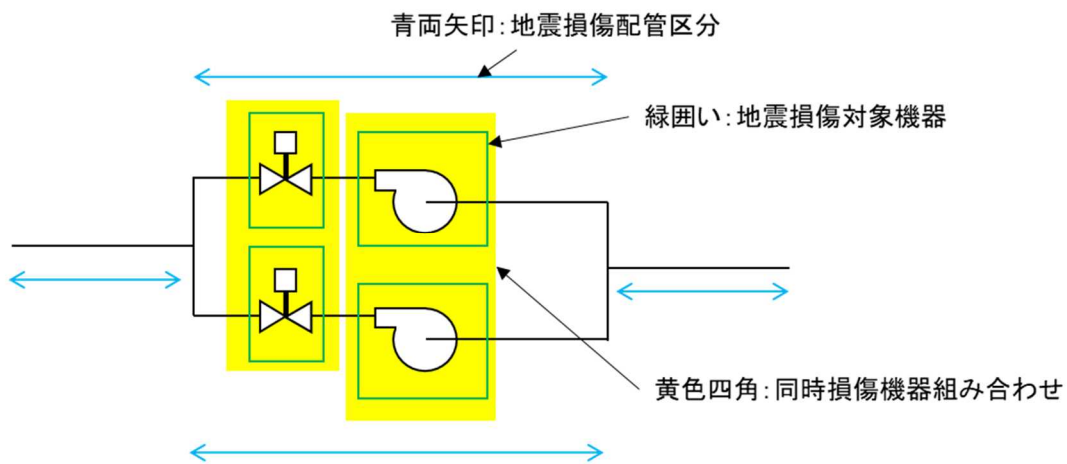
図 2 地震損傷対象機器の整理例
