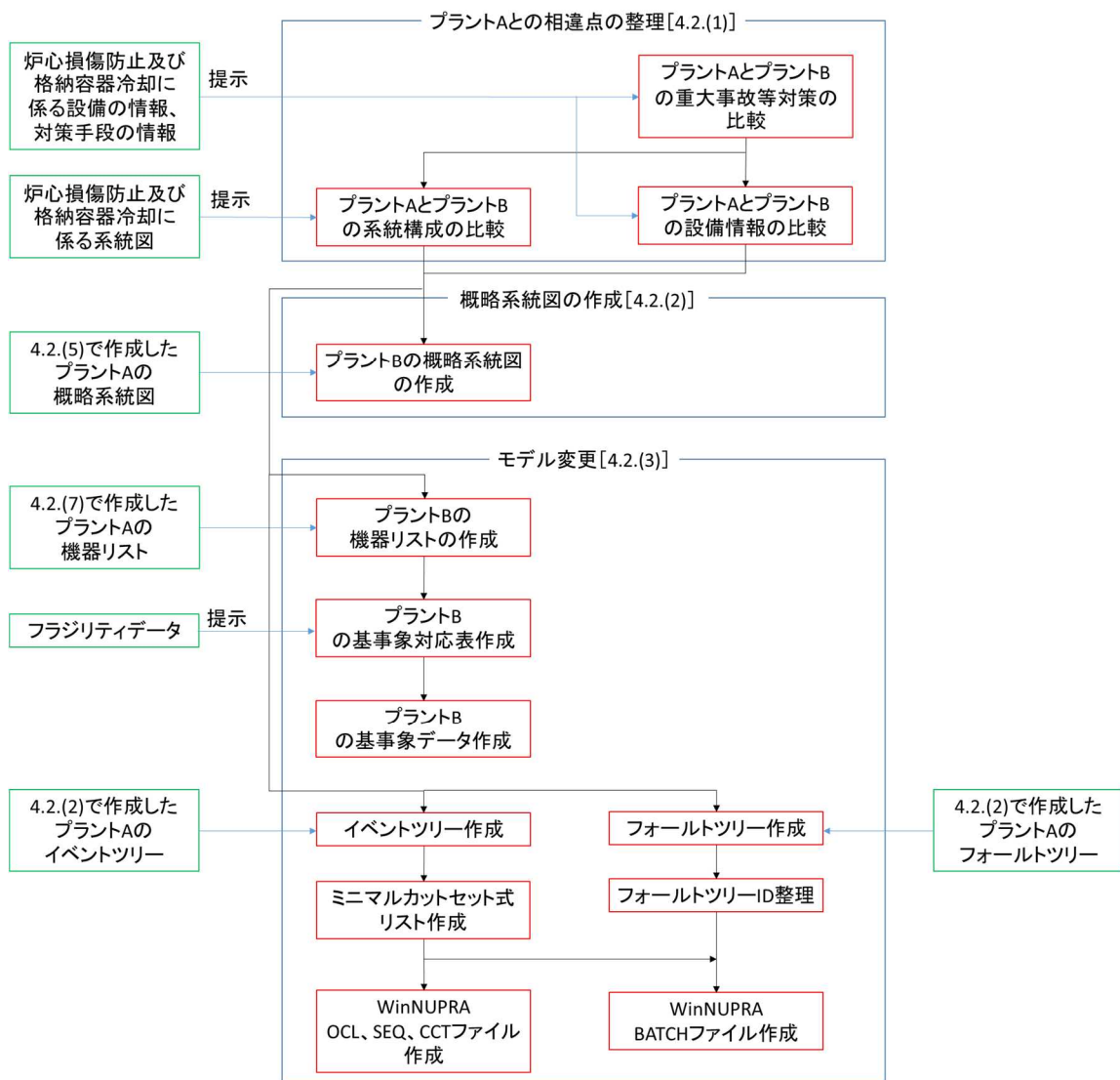
図 3 プラント B のモデル作成フロー
