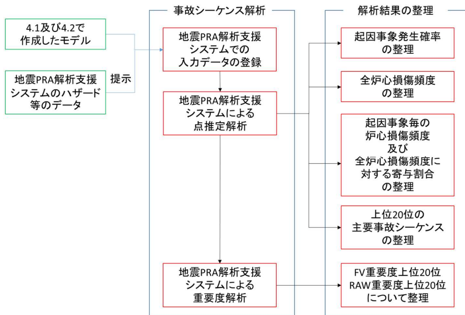
図 4 事故シーケンス解析のフロー
