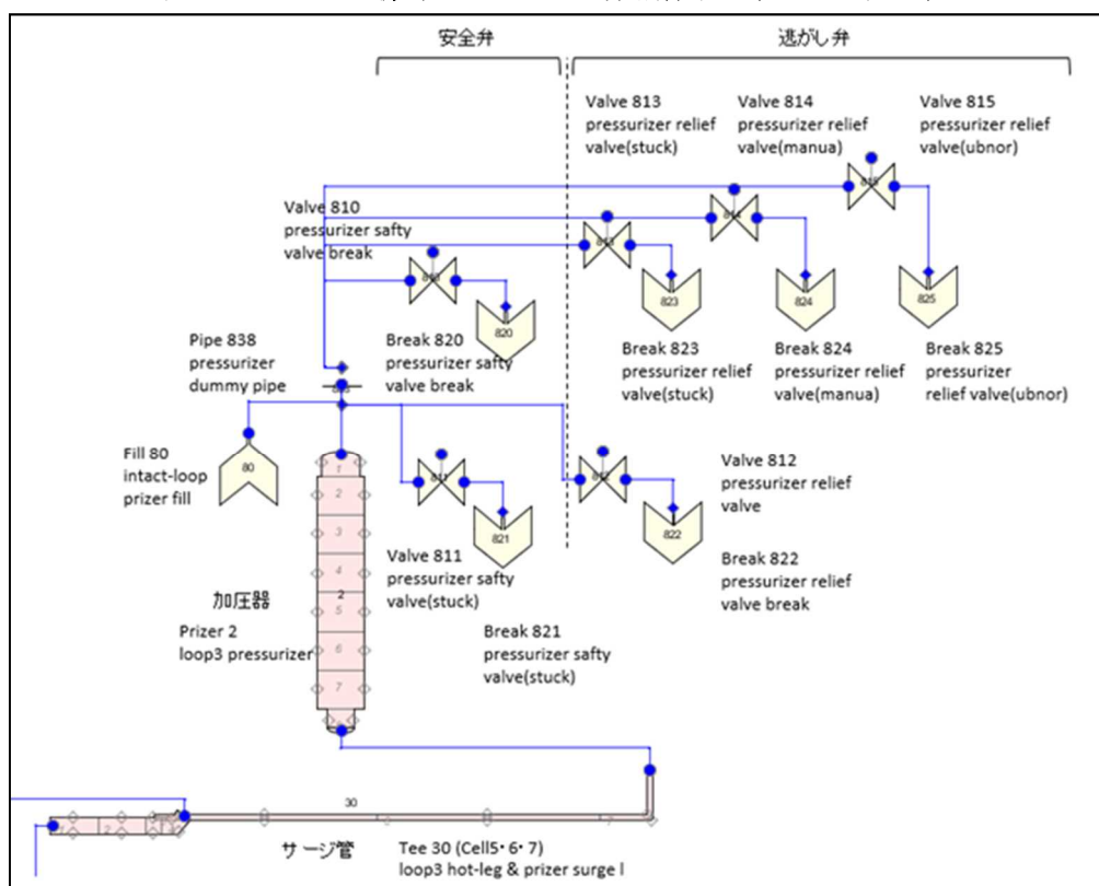
図2 加圧器関連のノード図 (SNAP 表示)
