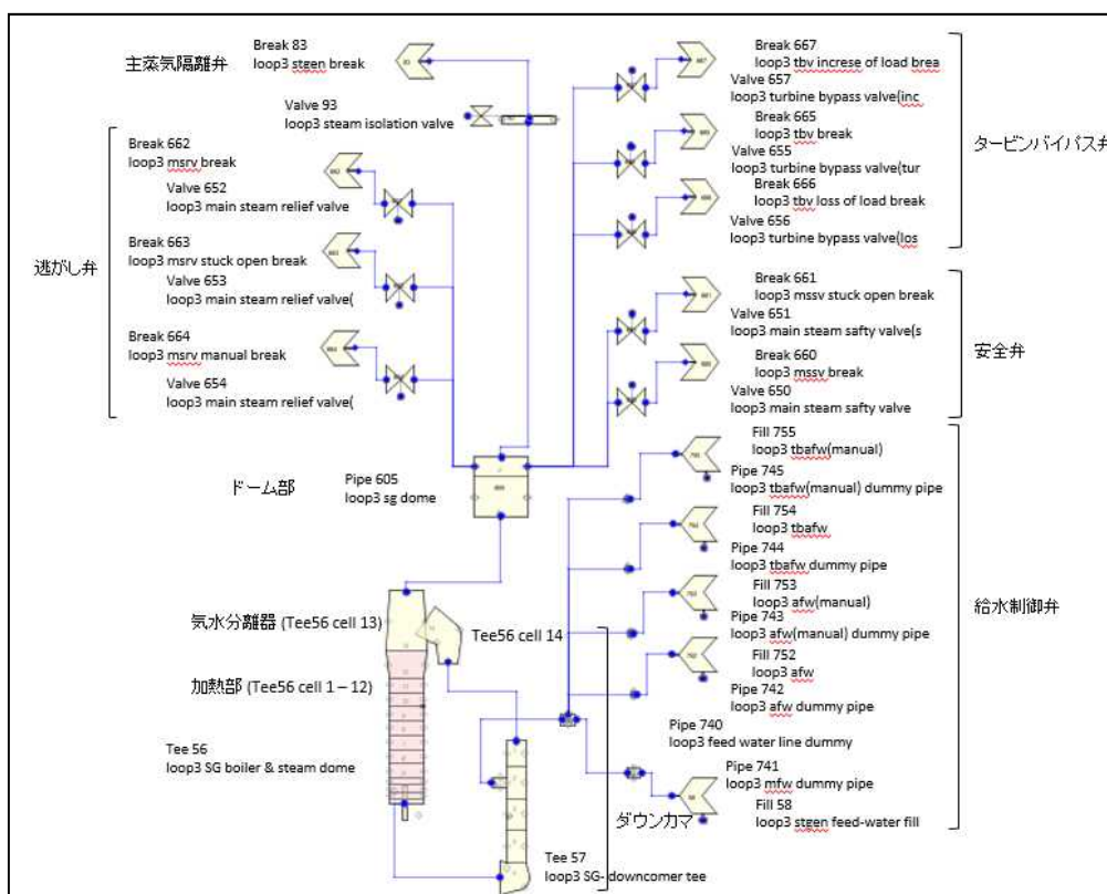
図 3 蒸気発生器（２次側）関連のノード図（SNAP 表示）
