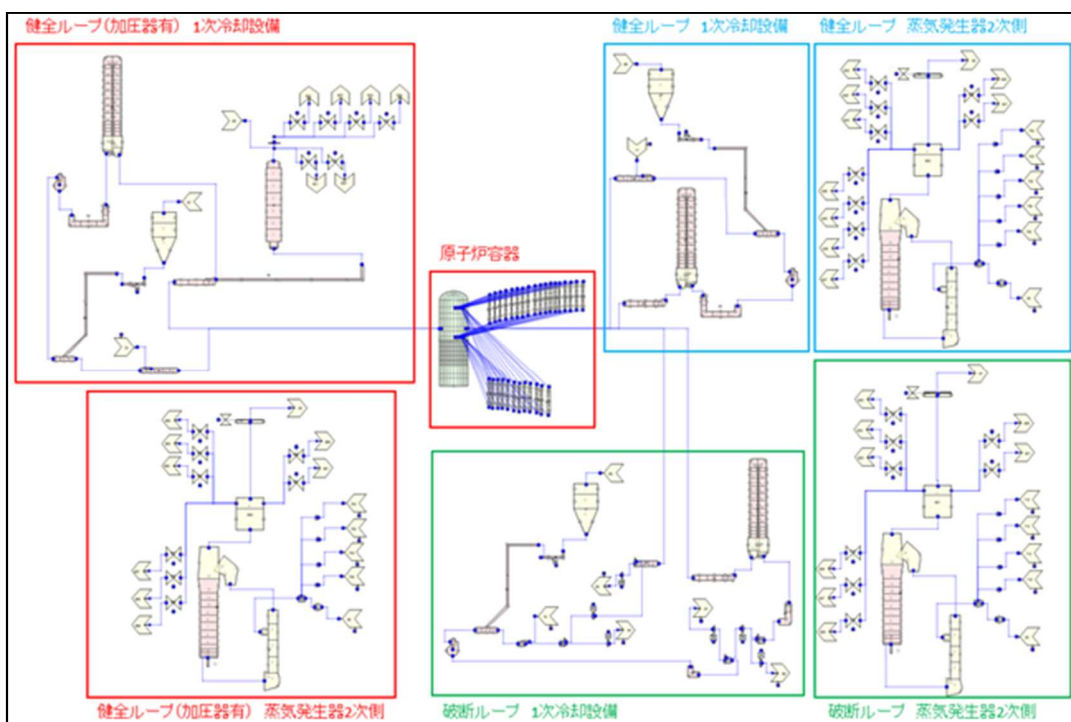
図1 TRACE 標準データの全体構成図 (SNAP 表示)
