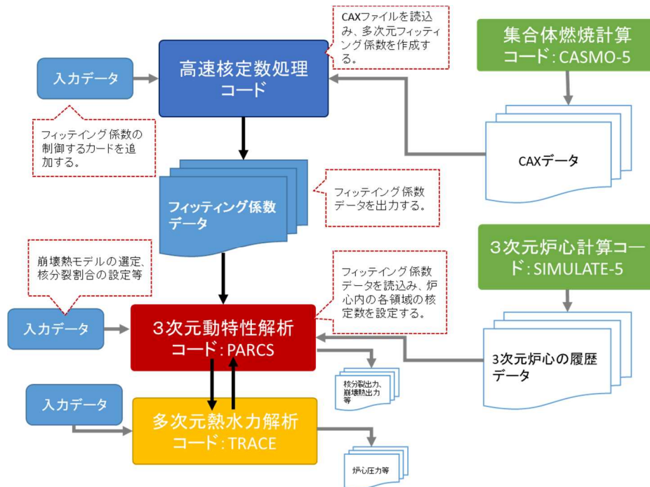
図 1 TRACE/PARCS コードを用いた核熱結合計算の流れ
