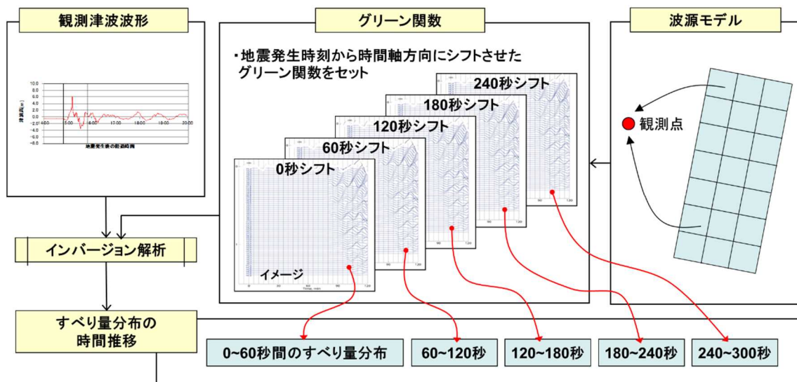
図 2 津波波源モデルにおけるすべり分布の経時変化の考慮の仕方(杉野他(2013)を一部修正)
