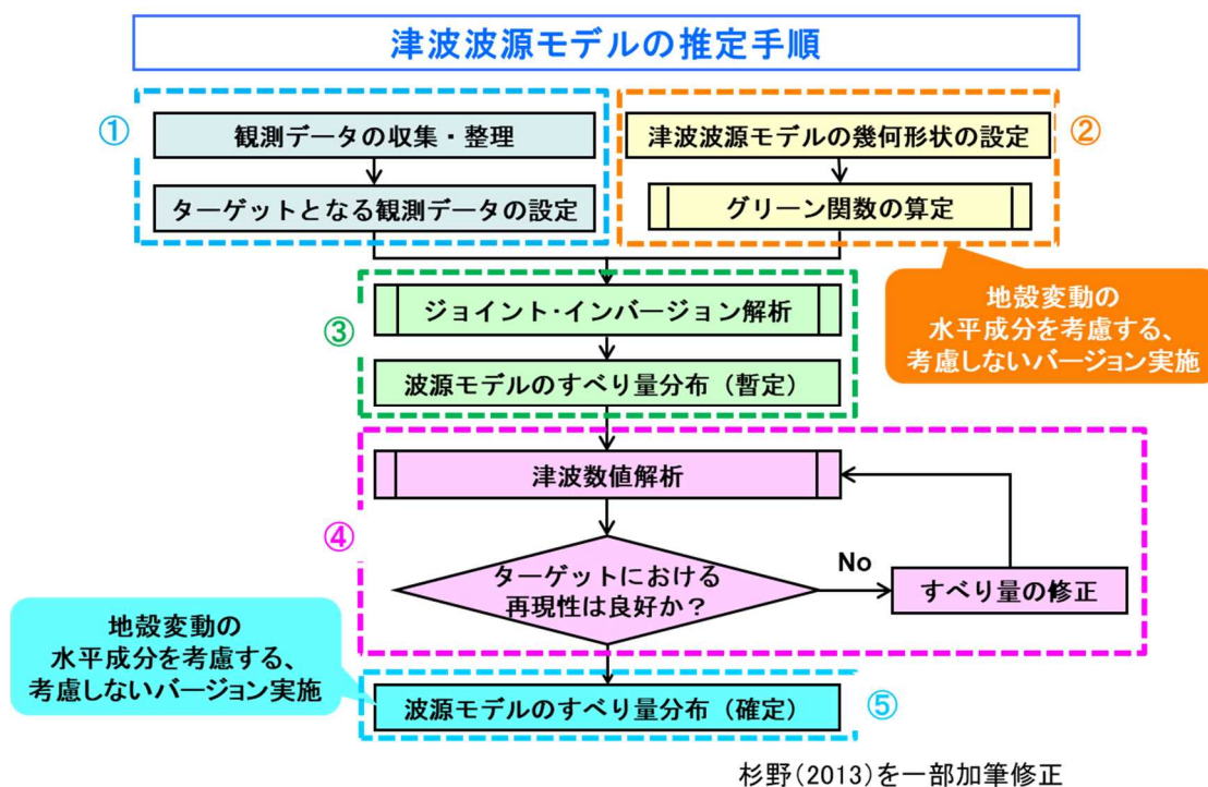
図 1 津波波源モデルの推定手順
