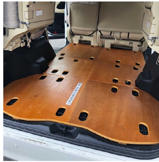
車内脱着式床板配置（6枚） （セカンドシート使用不可）
