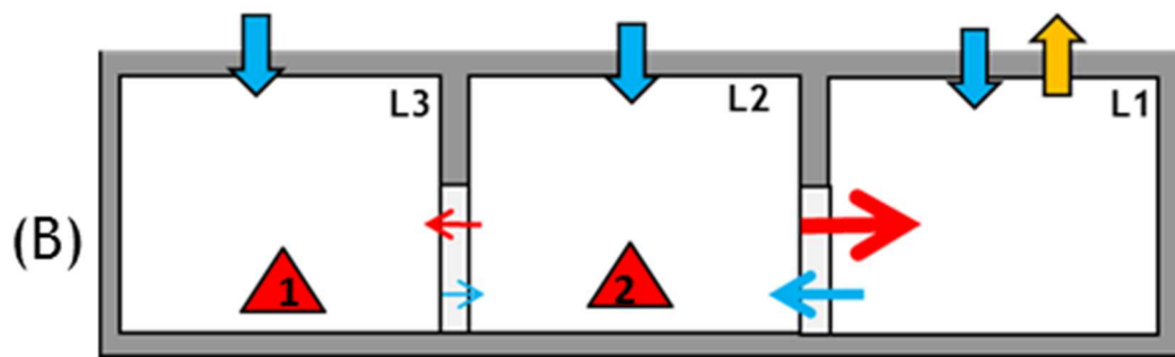
図 4.3.1 複数の火災源の試験体系
