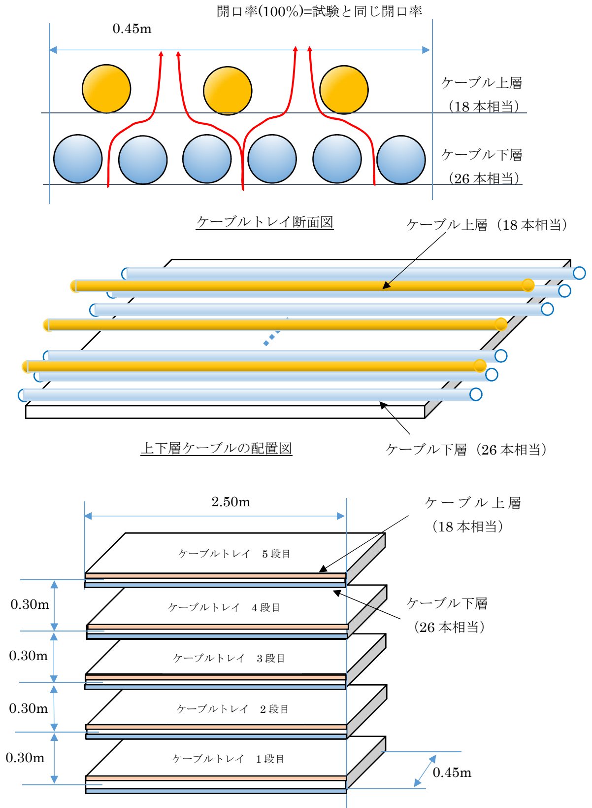
図 4.1.11 ケーブルトレイのモデル化方法
