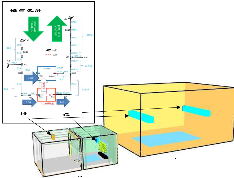
図 4.1.9 ベース解析モデルにおけるケーブル試験体の全体モデル図
