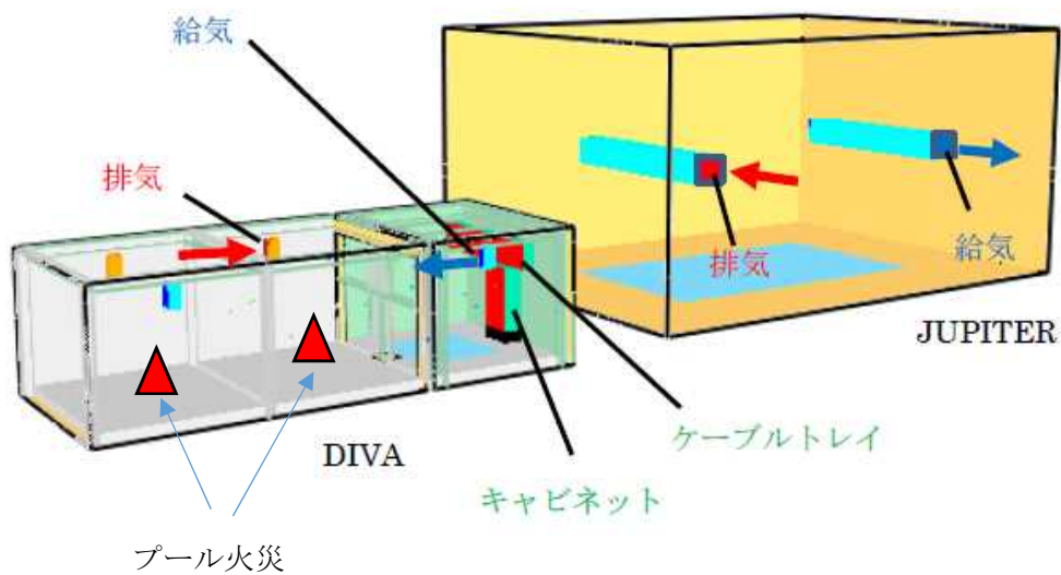
図 4.3.2 複数の火災源の解析モデルの全体概念図 (例)
