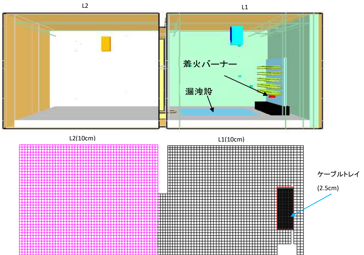
図 4.1.9 ベース解析モデルにおけるケーブル試験体の全体モデル図
