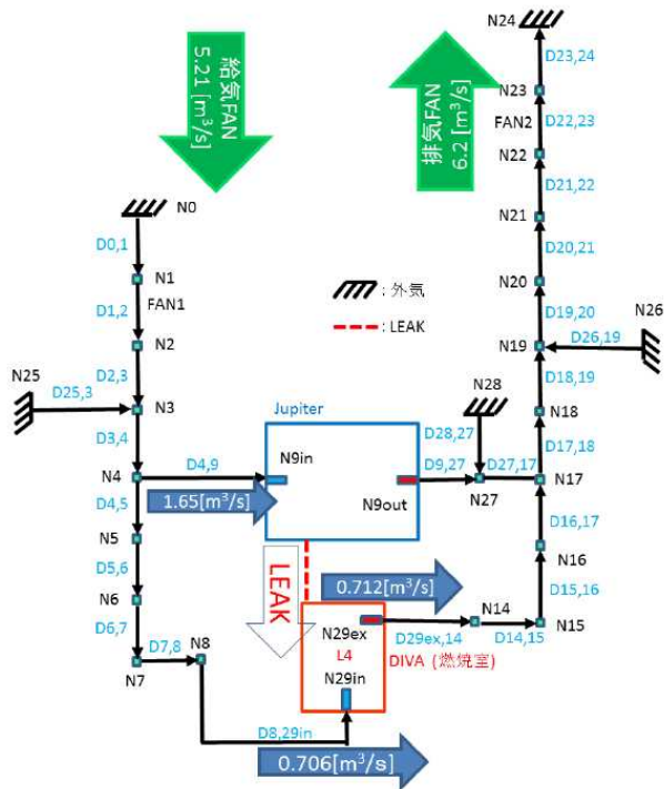
図 4.2.3 PRISME2 の消火試験体のベンチレーションネットワーク図
