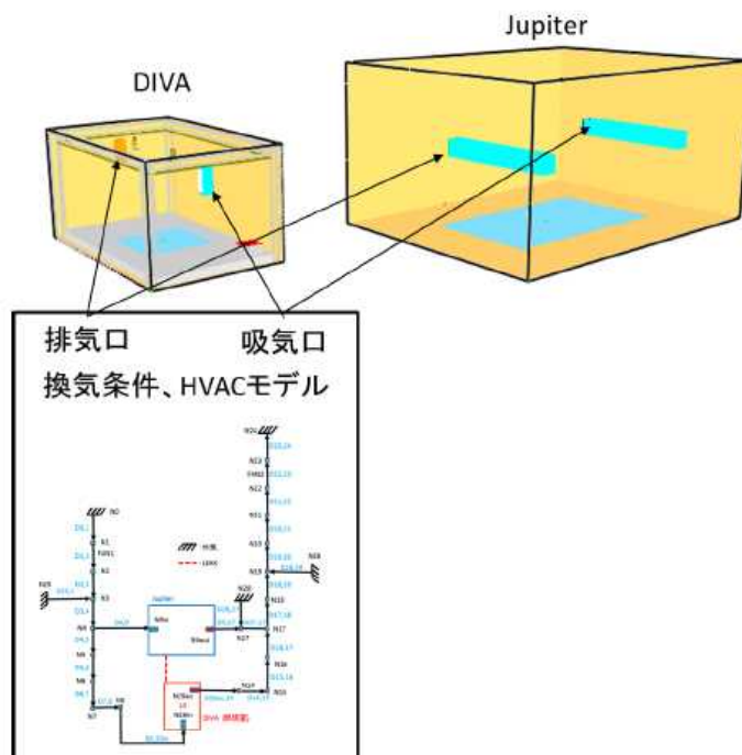
図 4.2.4 PRISME2 の消火試験体の解析モデルの全体図
