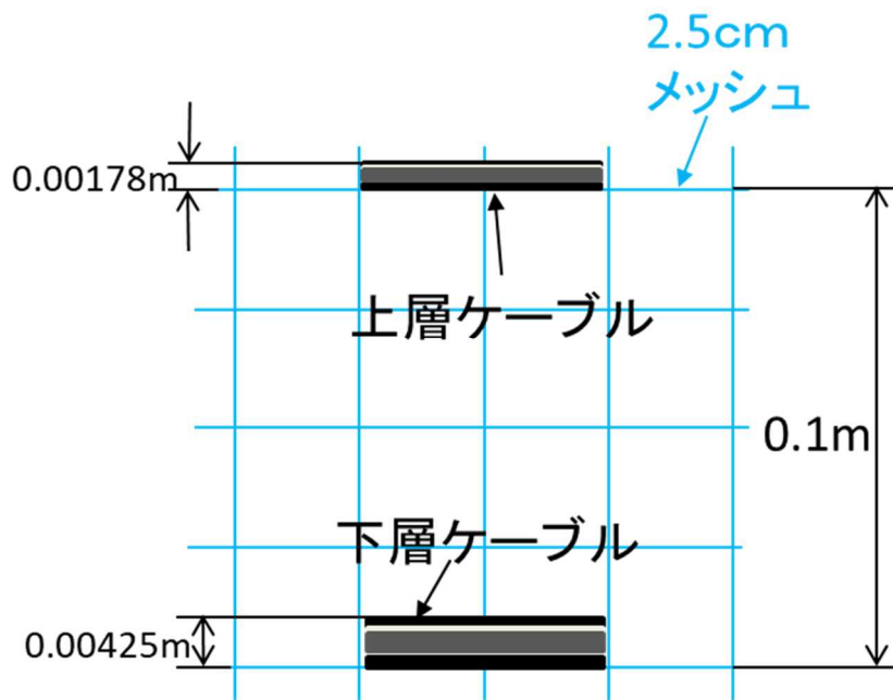
ケーブルトレイ部のメッシュ分割の方法
