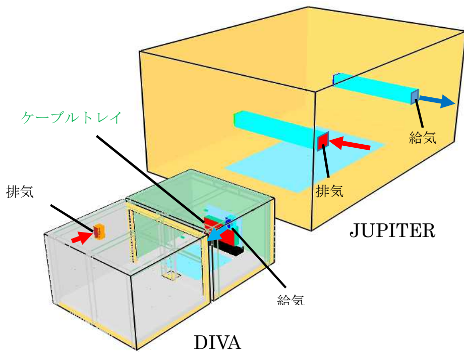
図 4.1.4 PRISME2 のケーブル試験体の全体モデル図
