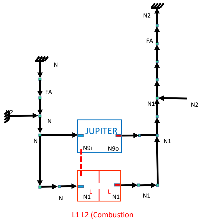
図 4.1.3 PRISME2 のケーブル試験体のベンチレーションネットワーク図
