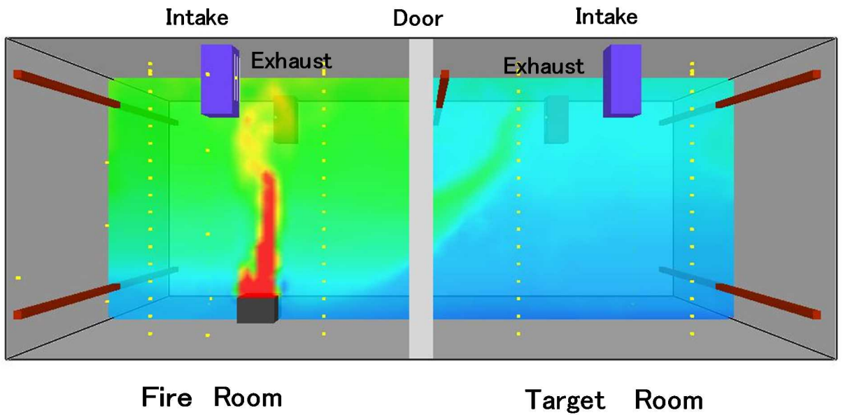
図 4.1.6 解析結果の温度分布出力例
