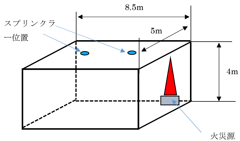
図 4.2.2 PRISME2 の消火試験体の概略形状
