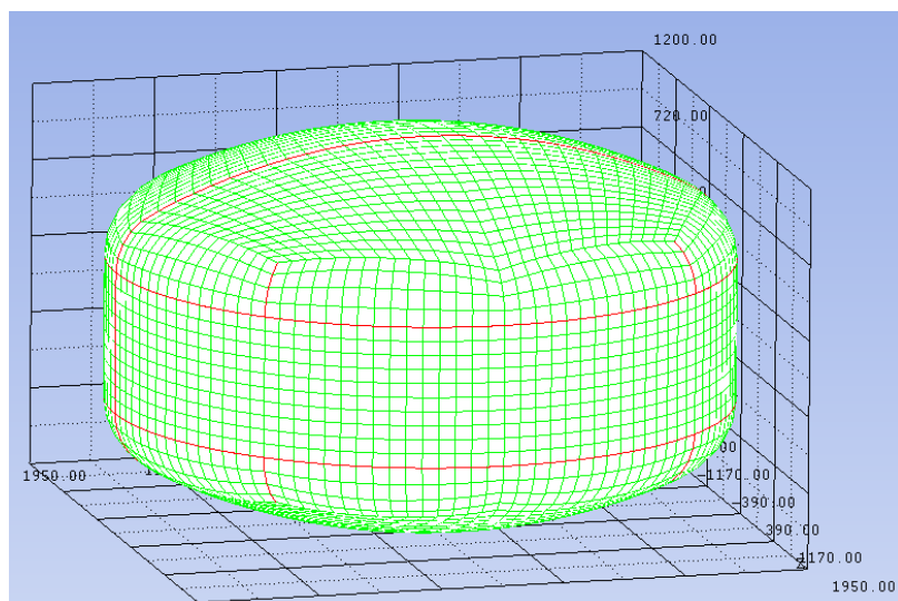
図2 排気ダクトの無い密閉された円筒型貯槽（単体）の形状データ （注：メッシュサイズについては、協議の上、決定する。）
