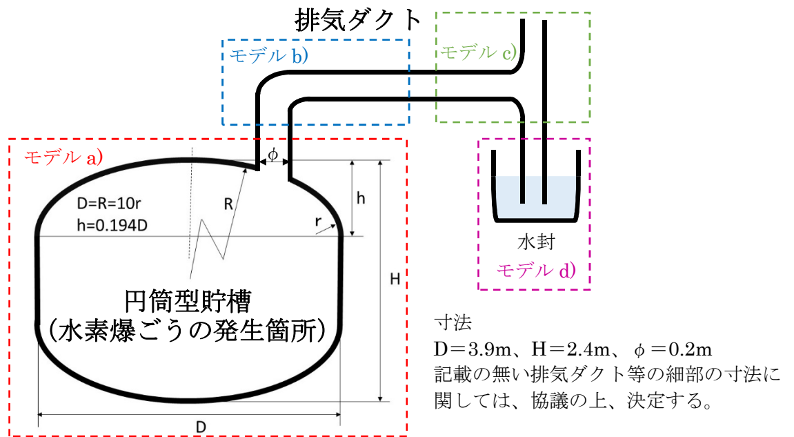
図1 円筒型貯槽及び排気ダクト（分岐や水封を含む。）の構造図
