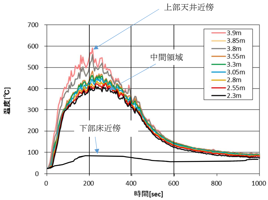
図 4.1-8 3次元火災コード(FDS)の解析結果例 (過渡変化)
