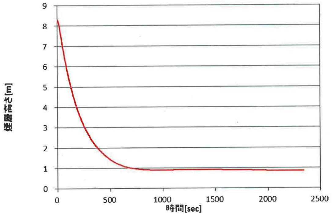
図 4. 1-4 ゾーンモデル火災コード(CFAST)の解析結果例 (煙層高さ)
