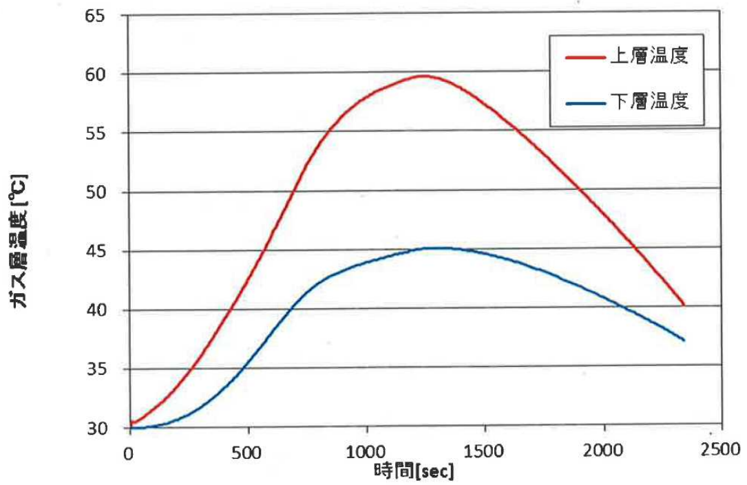
図 4. 1-5 ズーンモデル火災コード(CFAST)の解析結果例 (上層、下層温度)
