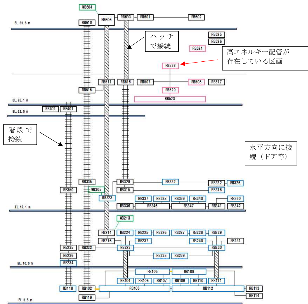
図 4.2-1 溢水シミュレーションコードを用いた建屋モデルの概念図
