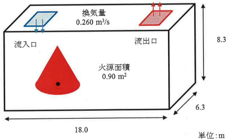
図 4. 1-3 ゾーンモデル火災コード(CFAST)の解析モデル例
