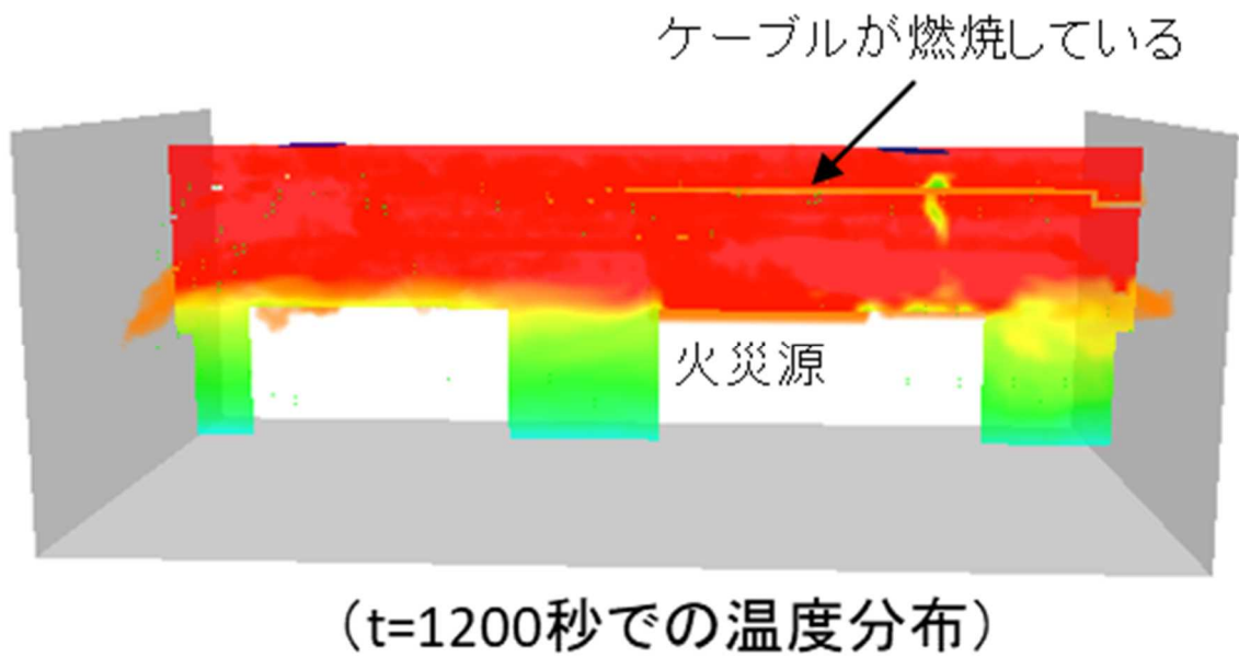
図 4.1-6 3次元火災コード(FDS)の解析モデル例
