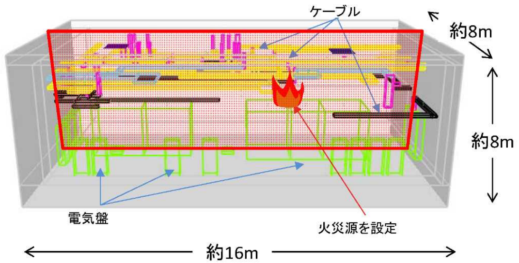
図 4.1-6 3次元火災コード(FDS)の解析モデル例
