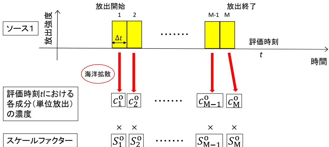
図 2. ソース 1 の時間変動。単位放出としたソース 1 を一定の時間間隔 ( \Delta t ) で分割し、それぞれを別種のトレーサとして拡散計算を行う。評価時刻 t における各成分の濃度 c_m^0 を記録しておき、それぞれにスケールファクター S_m^0 を適用する。
