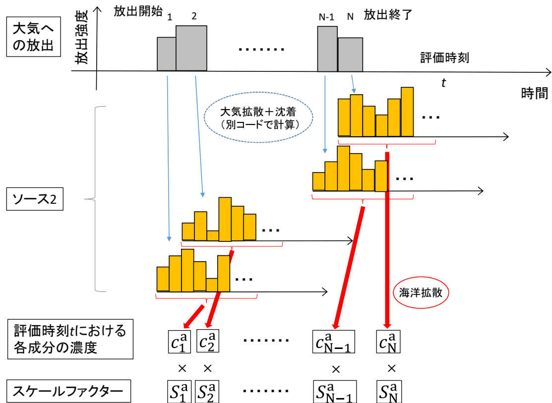
図3. ソース2の時間変動。大気への放出をあらかじめ時間により分割しておく、それぞれを別種のトレーサとして別コードで計算しておいた1時間ごとの海面への沈着フラックスをソース2として与え、拡散計算を行う。評価時刻 t における各成分の濃度 c_n^a を記録しておく、それぞれにスケールファクター S_n^a を適用する。
