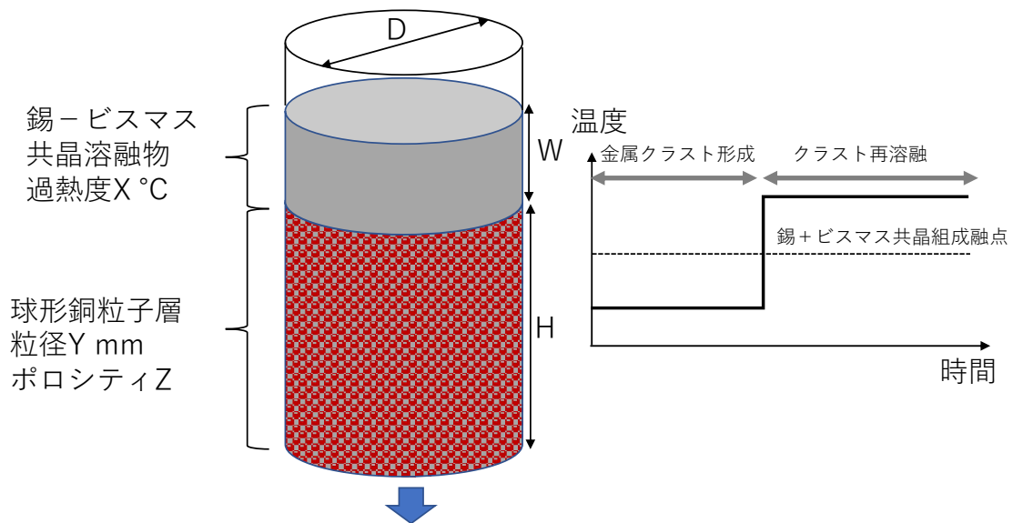
図4 REMELT ベースコードのための REMCOD-3 実験体系
