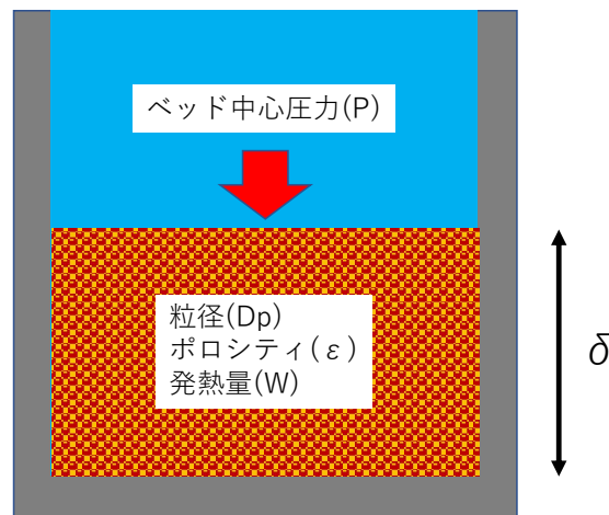
図 5 粒子層限界熱流束体系
