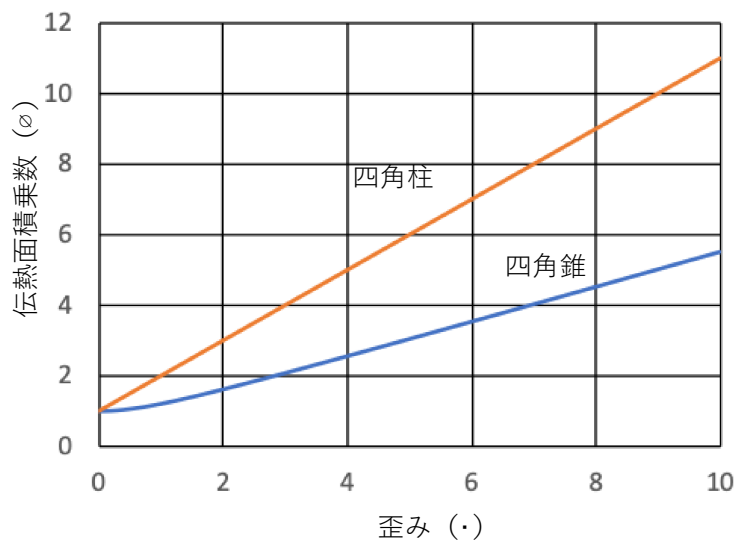
図3 表面線歪みと伝熱面積乗数の例
