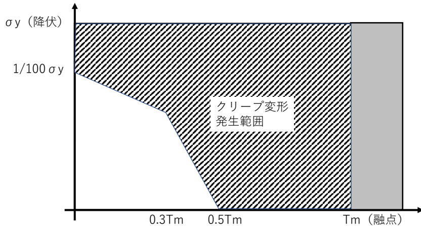
図2 クラスト伝熱面積増加温度-応力マップの例
