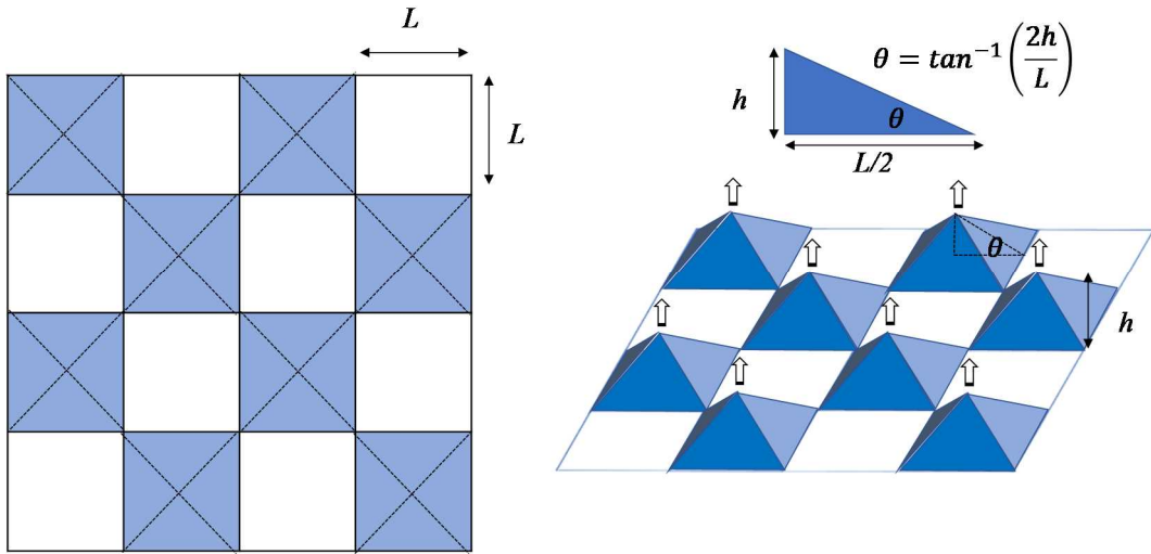
図1 沸騰によるクラスト伝熱面積増加モデル概念（変形が四角錐の場合）
