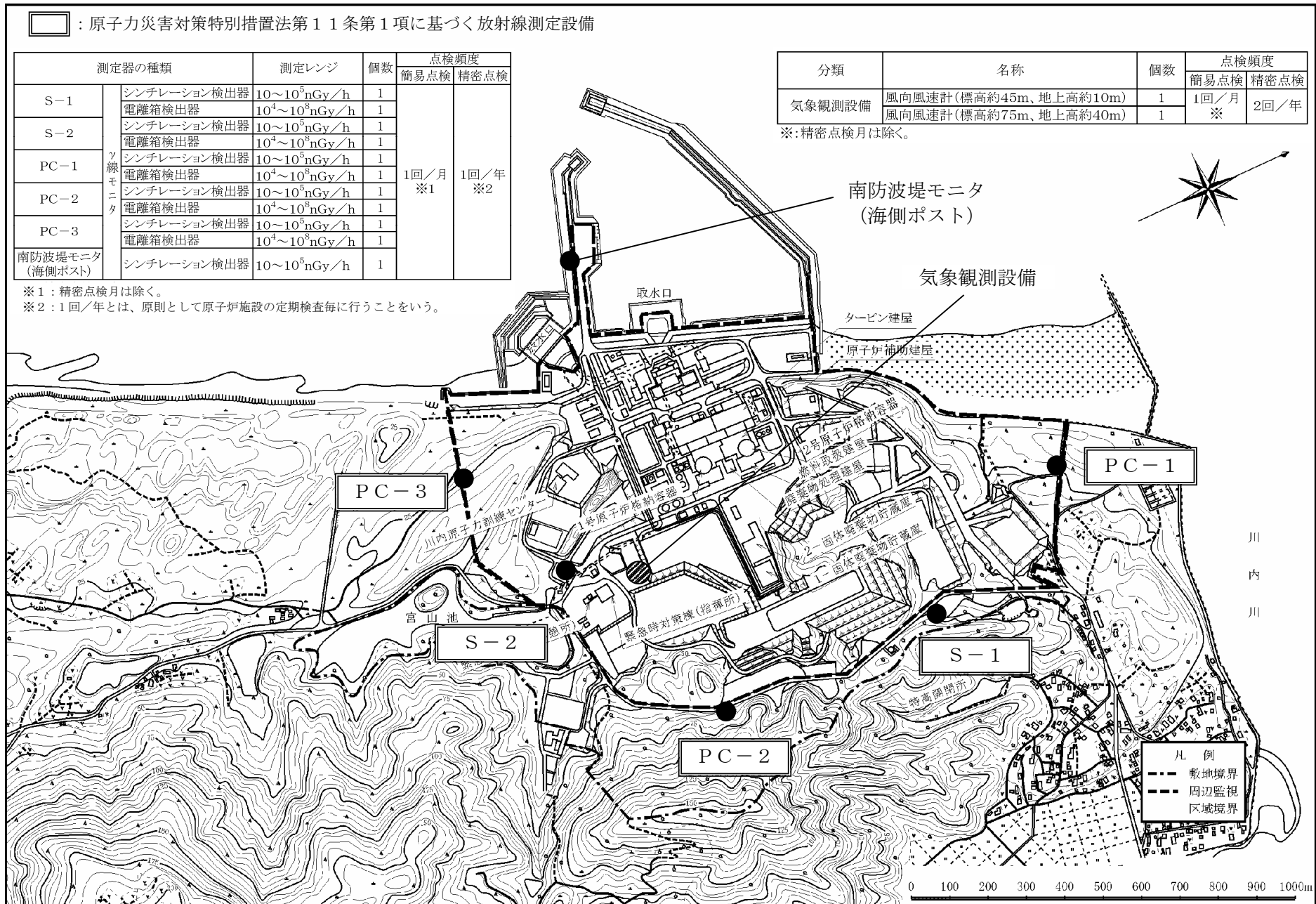
別図 3-2 発電所敷地境界付近の放射線測定設備等
