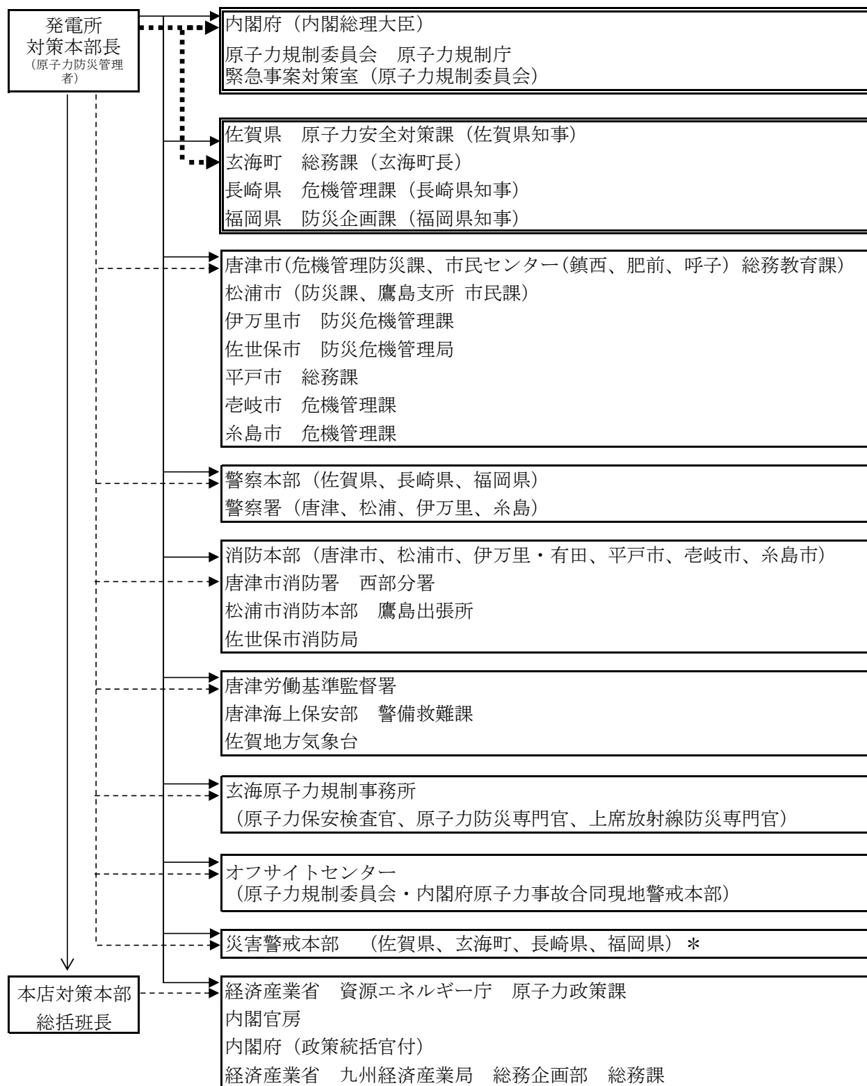
別図 2-4 (1) 原災法第 10 条第 1 項に基づく通報先 (発電所内での特定事象発生時の通報先)
