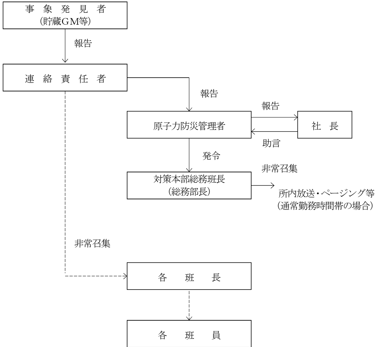
別図2-6 備蓄センターにおける緊急時態勢発令と緊急時対策要員の非常召集連絡経路
