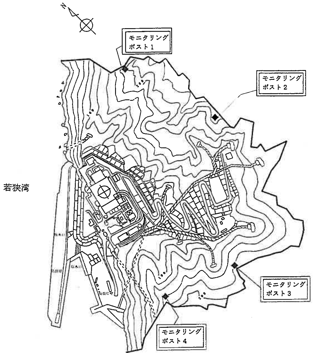
別図 2-3-10 もんじゅ敷地境界付近の放射線測定設備
