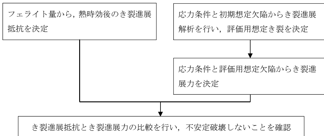
図4 熱時効評価の流れ
