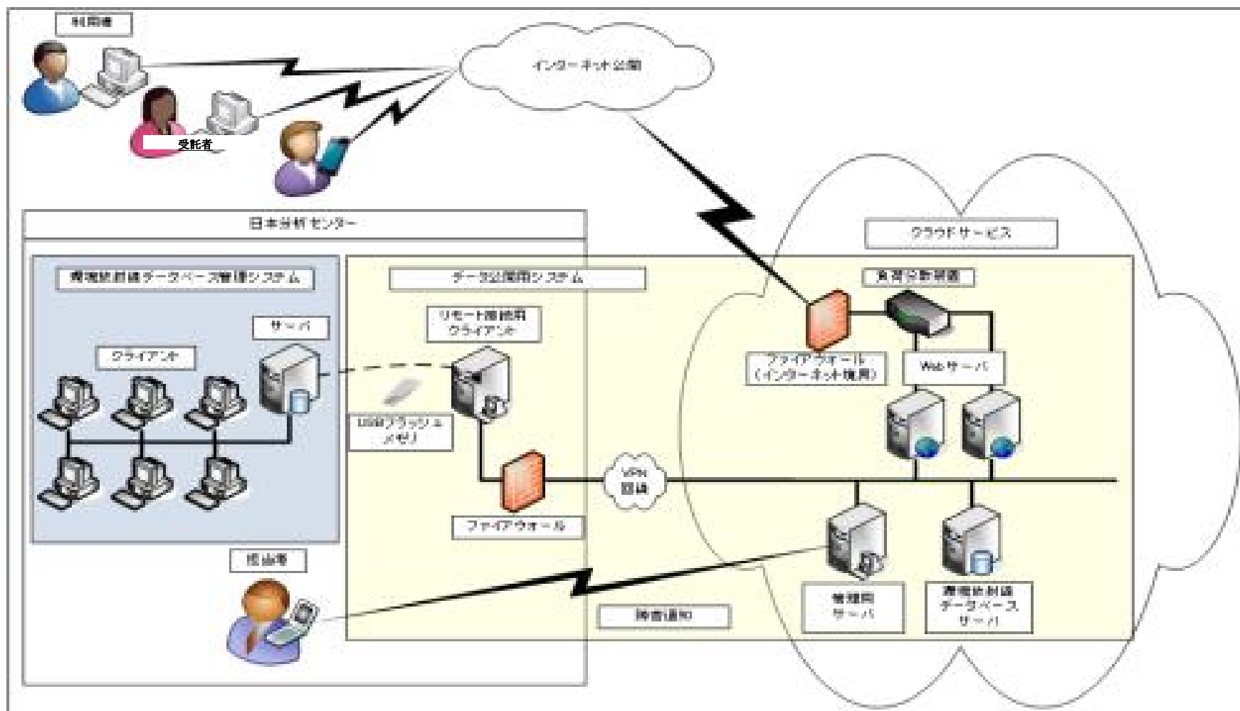
環境放射線データベース管理システム及びデータ公開用システムの構成図
