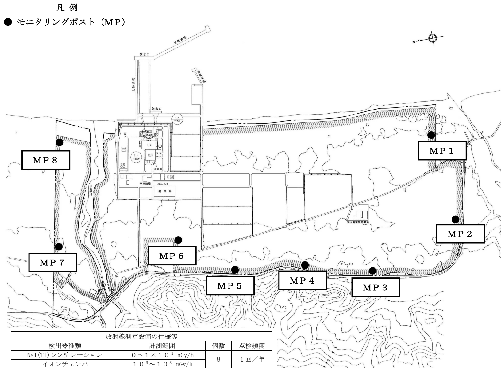
別図 2-1-1 発電所敷地周辺の放射線測定設備の配置
