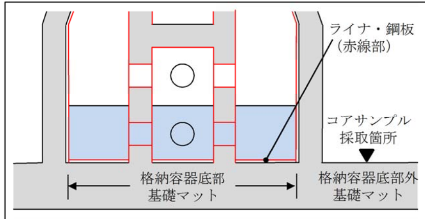
図 4. 1. 1-1 格納容器底部基礎マット概要図
