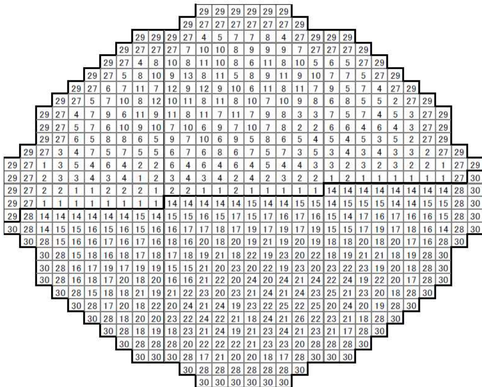
図 4 TRACE/PARCS の Ringhals-1 号機の炉心分割図(例)
