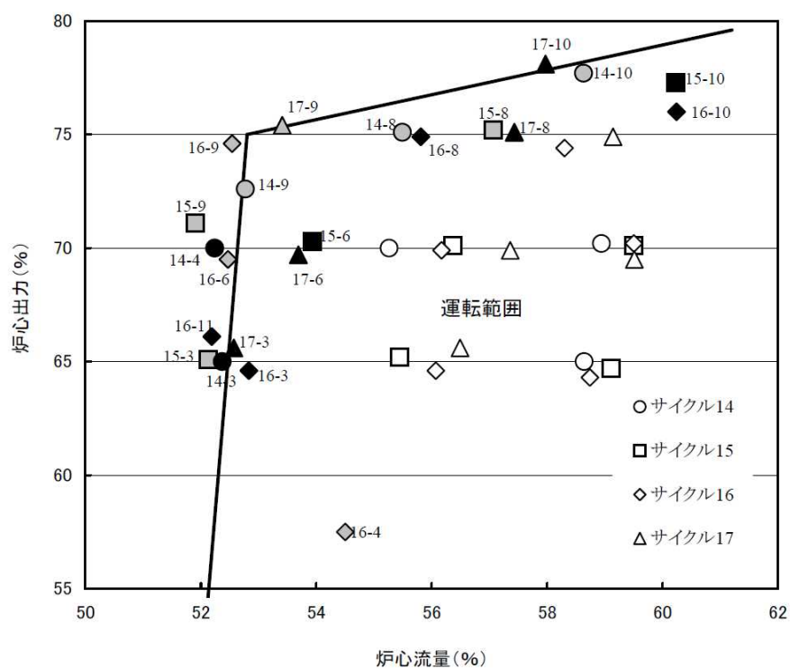
図 2 Ringhals-1 号機安定性試験点
