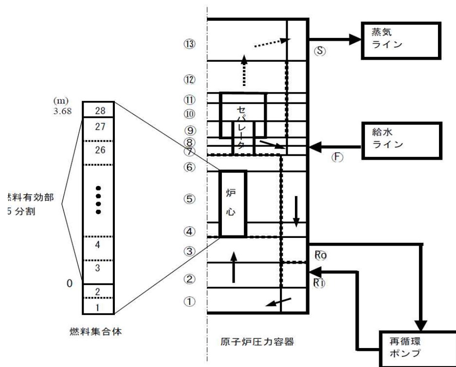
図5 Ringhals-1号機安定性試験解析のノード分割例
