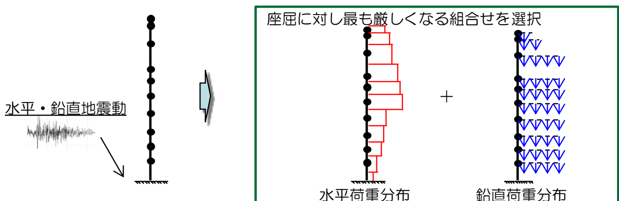
図1 質点系解析モデルと応答分布の算出（例）
