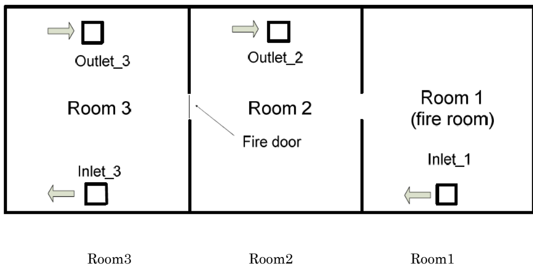
図 4.1.4 PRISME2 試験体(CFS-5)の水平断面図
