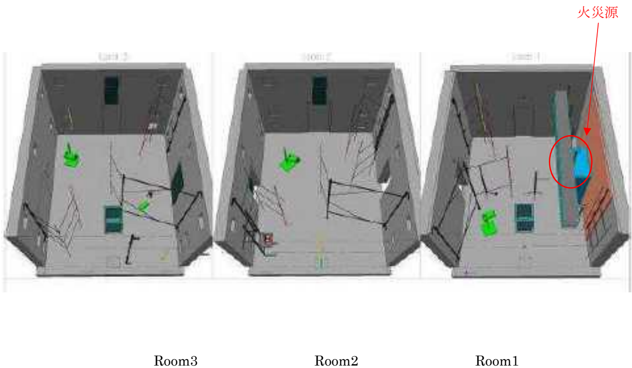
図 4.1.3 PRISME2 試験体(CFS-5)の3次元鳥瞰図
