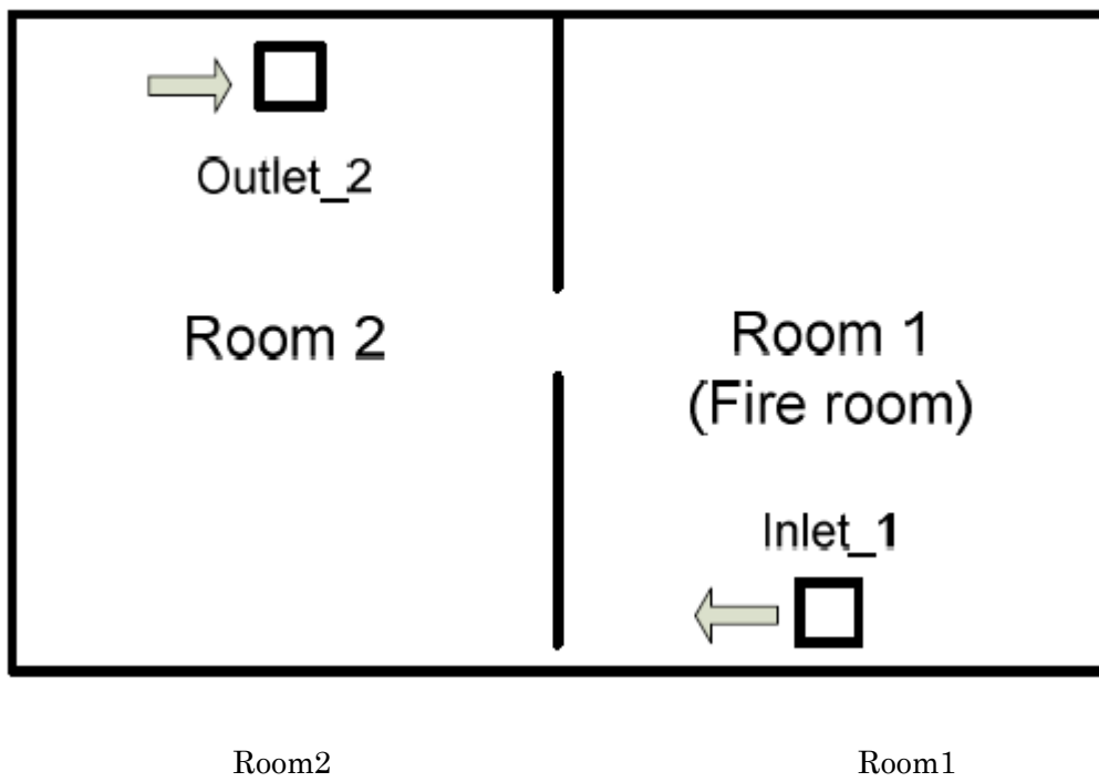
図 4.1.2 PRISME2 試験体(CFS-1)の水平断面図
