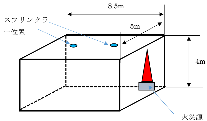
図 4.2.2 PRISME2 試験体(FES-3)の概略形状
