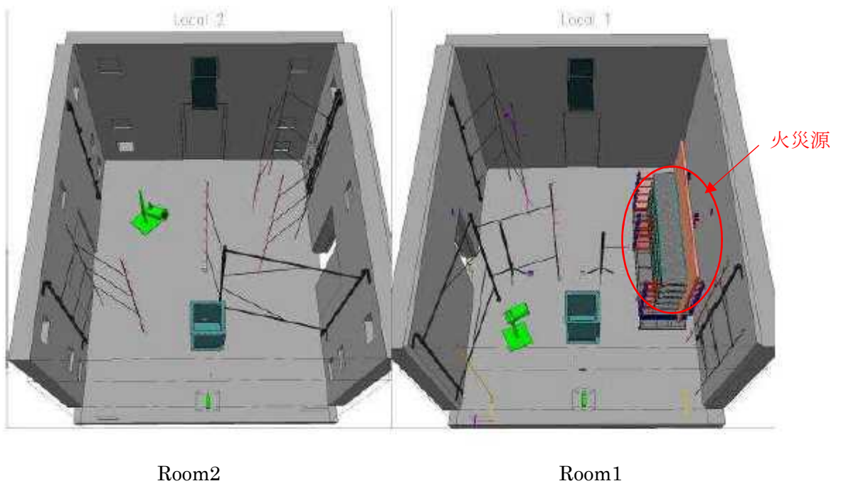
図 4.1.1 PRISME2 試験体(CFS-1)の 3 次元鳥瞰図
