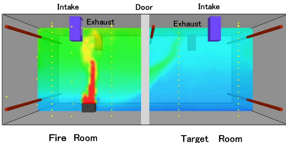
図 4.1.7 解析結果の温度分布出力例
