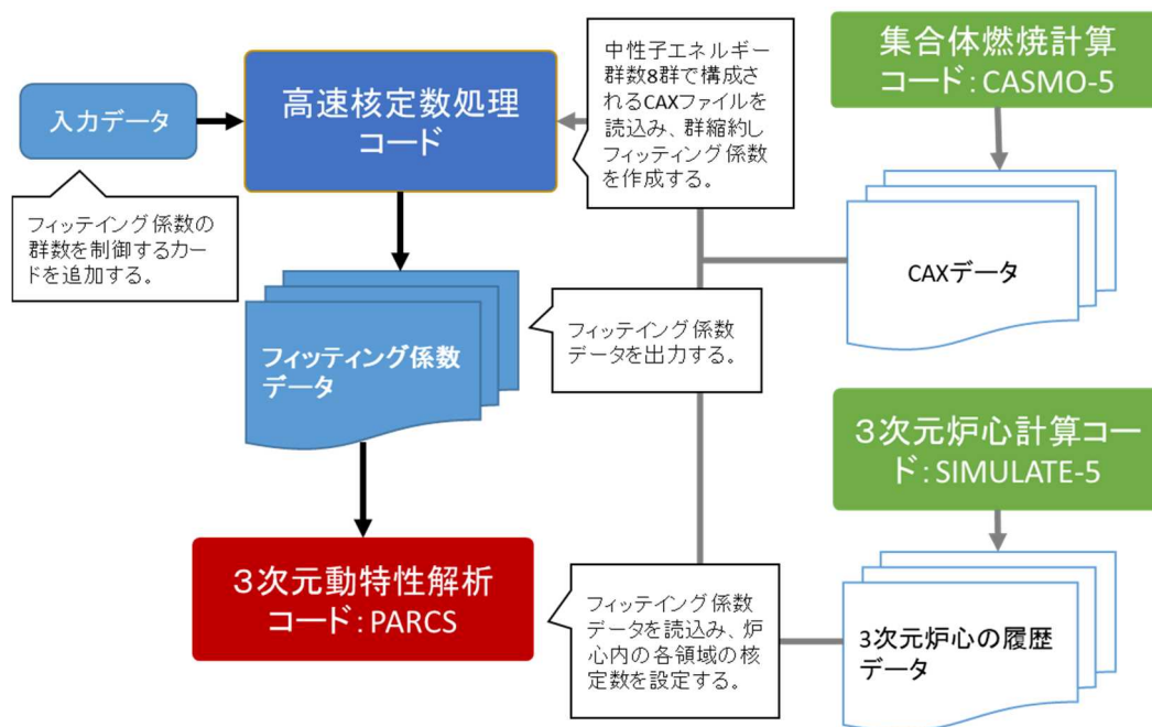
図1 PARCSコード用核定数フィッティング係数の処理の流れ
