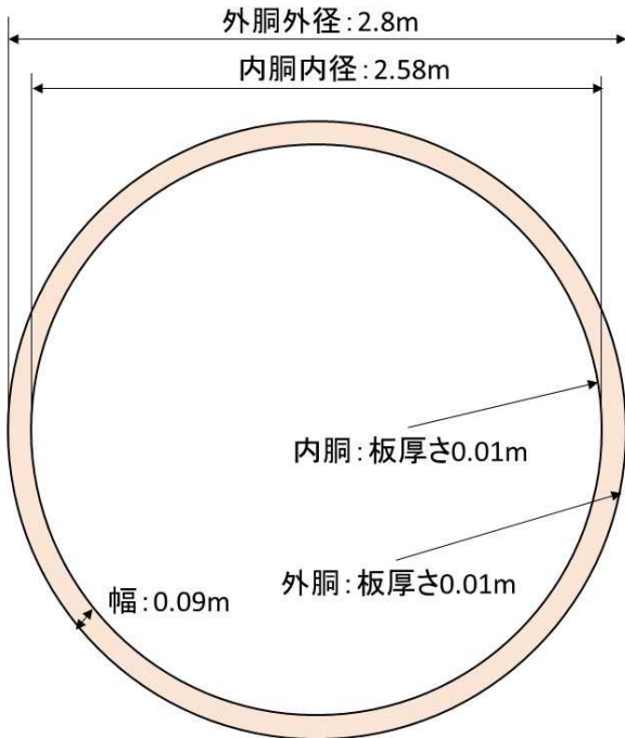
(1) 気相部の平面
