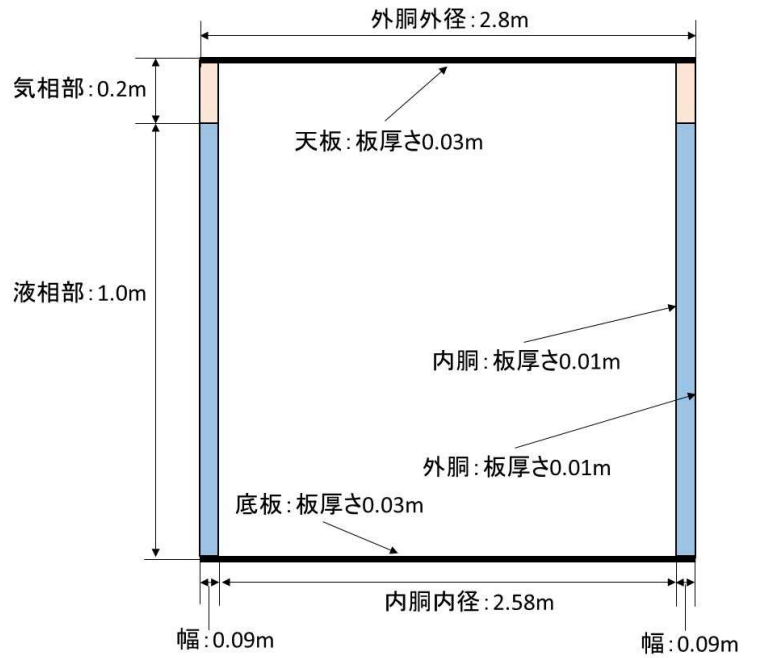
(2) 気相部＋液相部の断面
