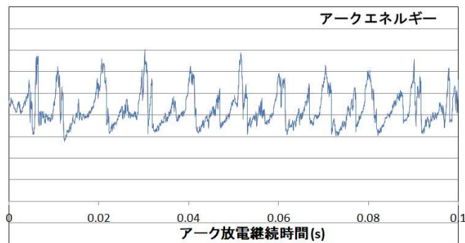
図 1 アークエネルギーの推移の一例
