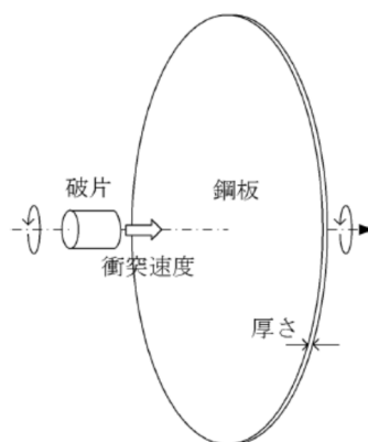
図3 HEAF により生じた電源盤破片の衝突解析の模式図
