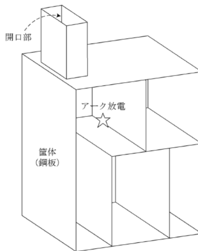
図2 実電源盤に対する HEAF 試験の再現解析の一例
