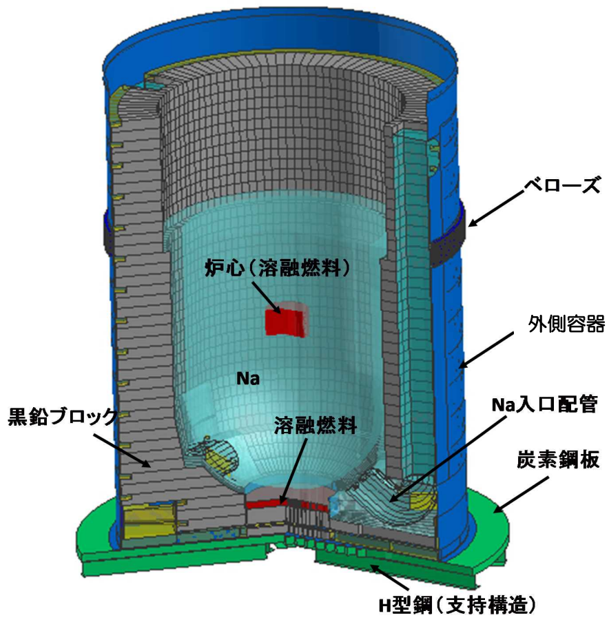
図1 解析モデル (昨年度モデル)
