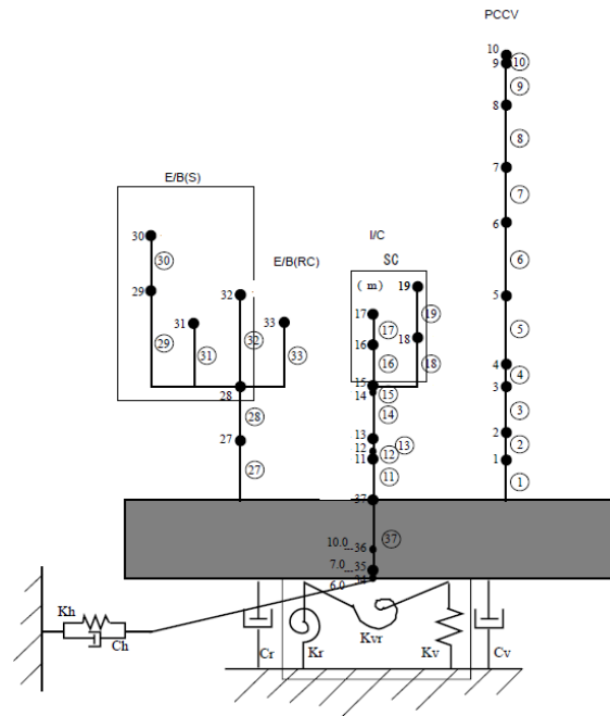
図2 地震応答解析モデルのイメージ (PWR) 4)
