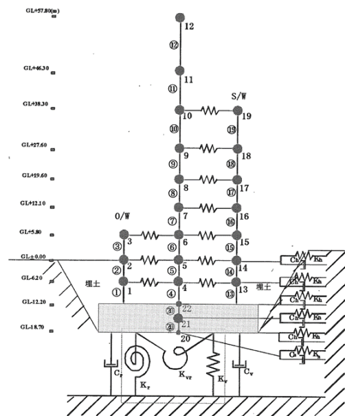
図1 地震応答解析モデルのイメージ (BWR) 3)
