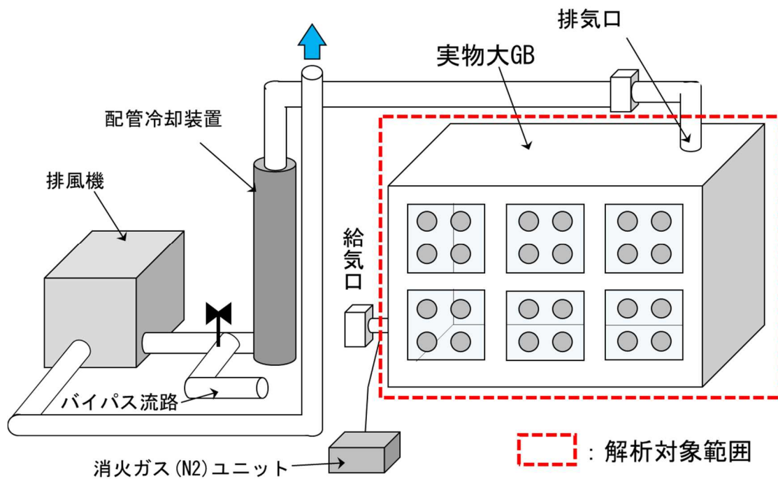
図 1 GB 内火災試験装置の模式図
