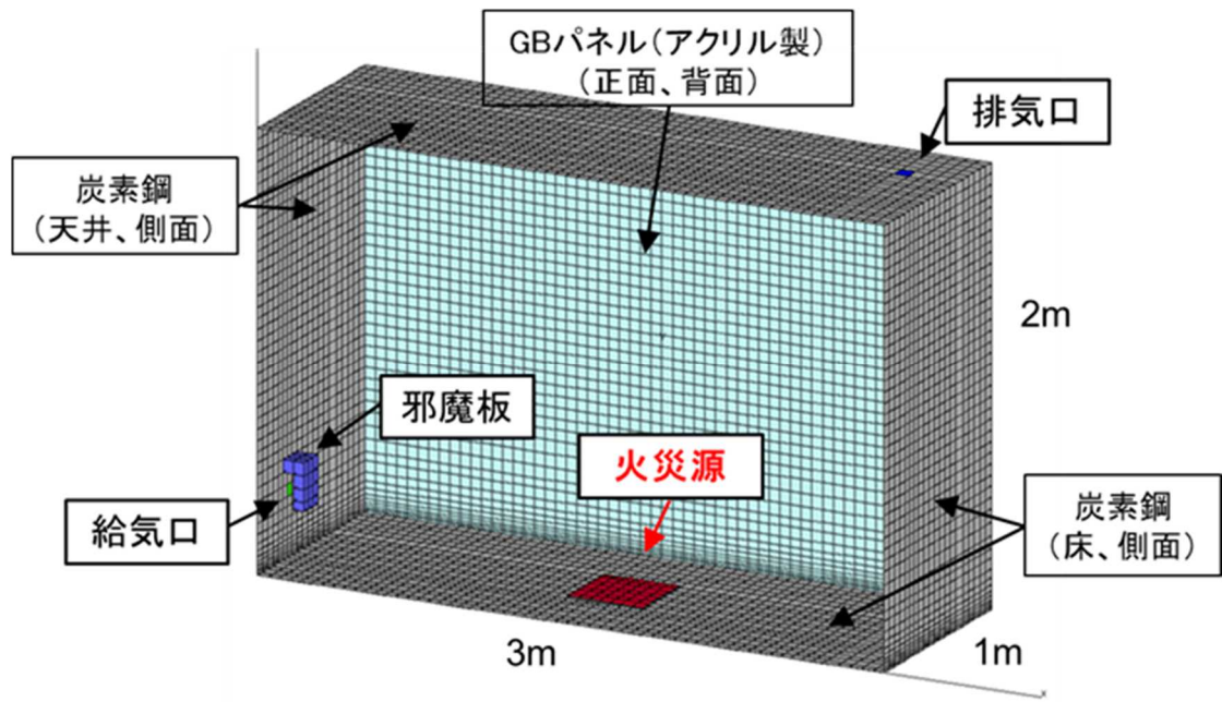
図2 基本ケースの解析体系
