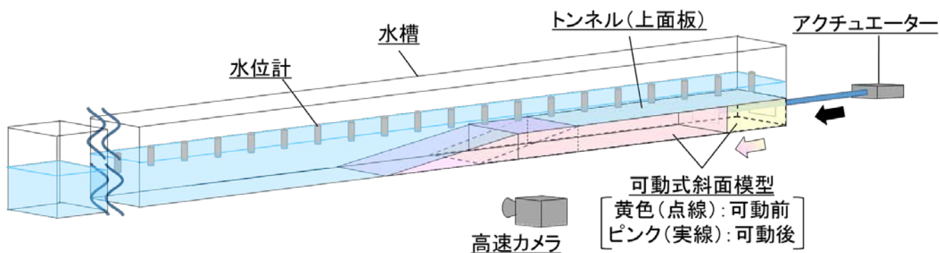
図 1 水理実験の概要
