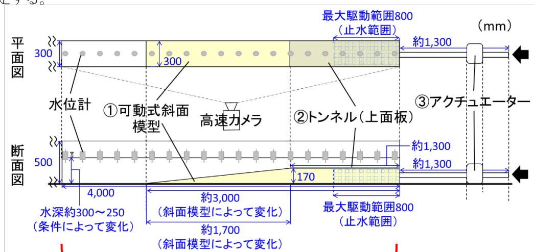
図 3 実験で使用する水理実験装置の概要案
