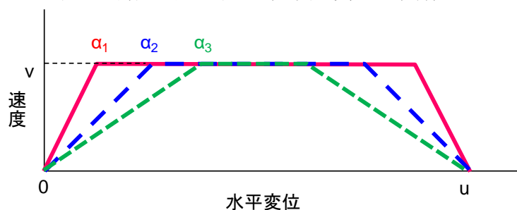
図 5 海底地形の動き (加速度が異なる場合)
