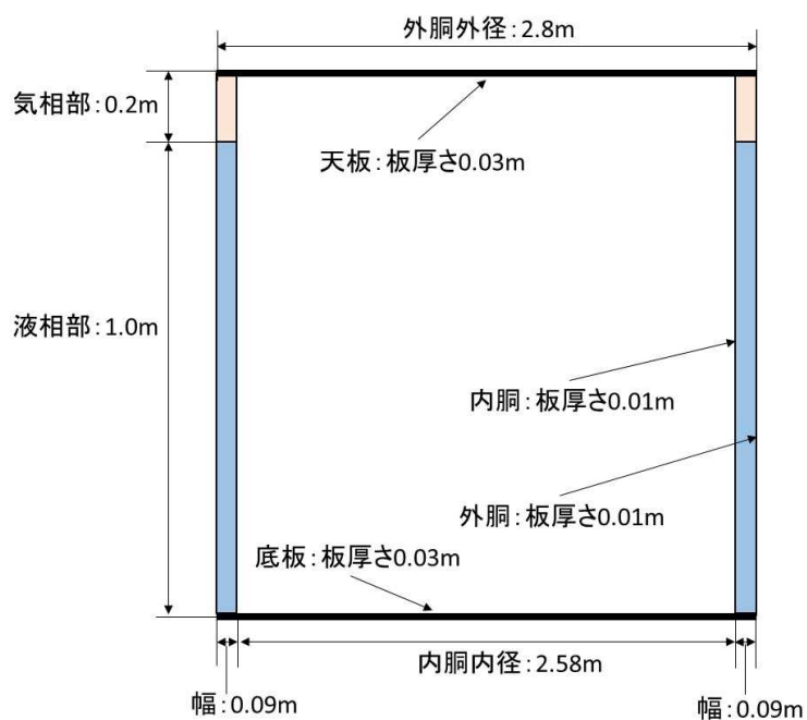
(2) 気相部＋液相部の断面
