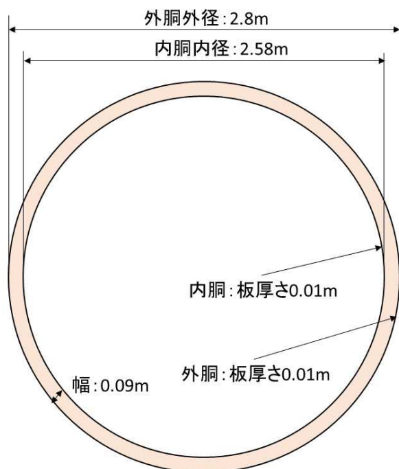
(1) 気相部の平面
