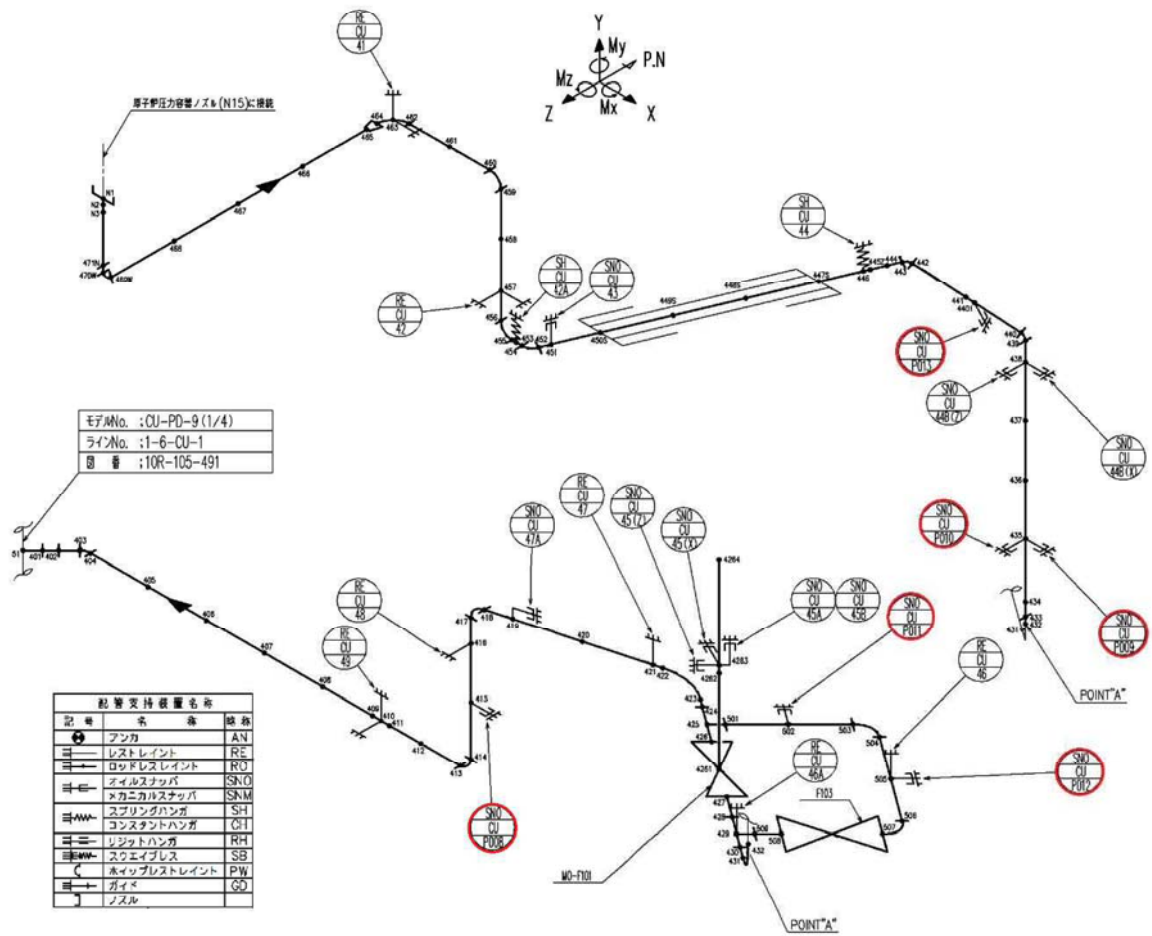
図 15 (2/4) 補正工認等による耐震補強実施箇所【原子炉冷却材浄化系】
