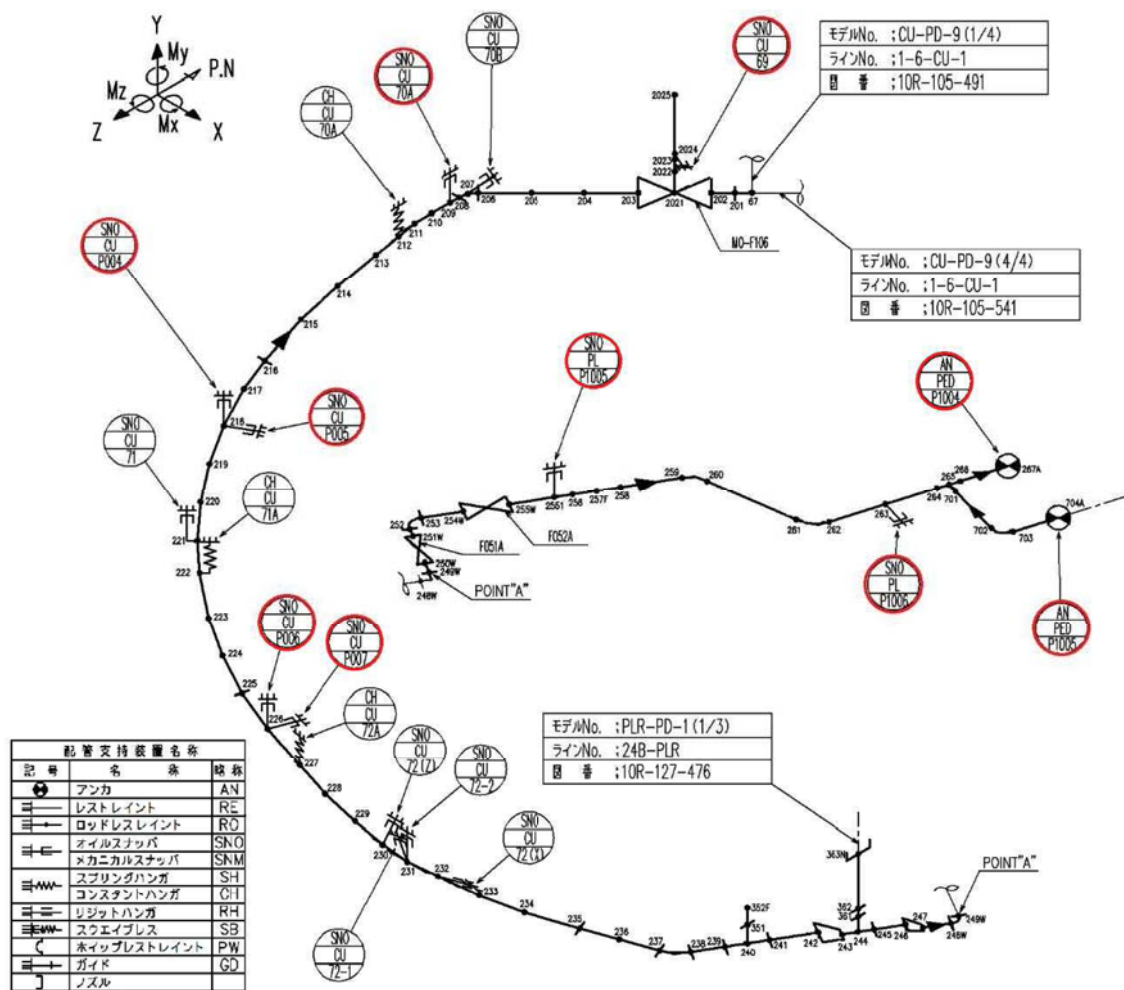
図 15 (3/4) 補正工認等による耐震補強実施箇所【原子炉冷却材浄化系】
