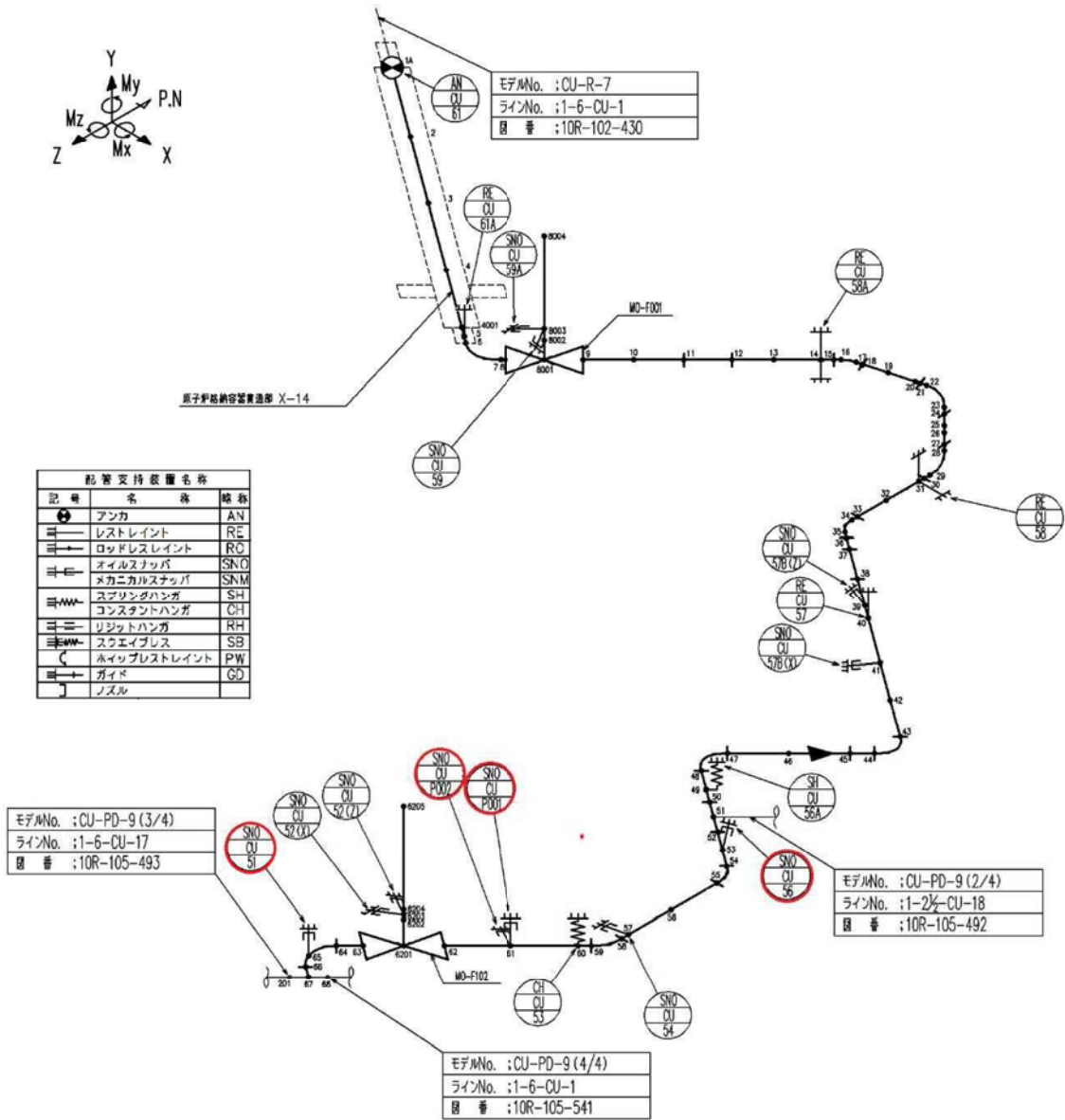
図 15 (1/4) 補正工認等による耐震補強実施箇所【原子炉冷却材浄化系】
