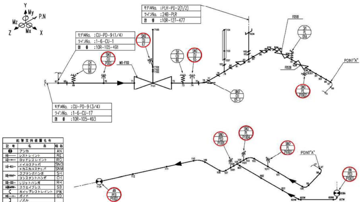
図 15 (4/4) 補正工認等による耐震補強実施箇所【原子炉冷却材浄化系】
