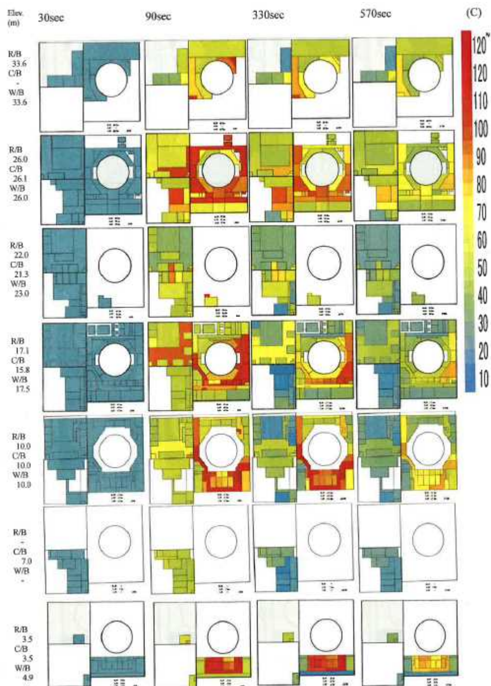
図 4.2-3 区画の可視化の作成例
