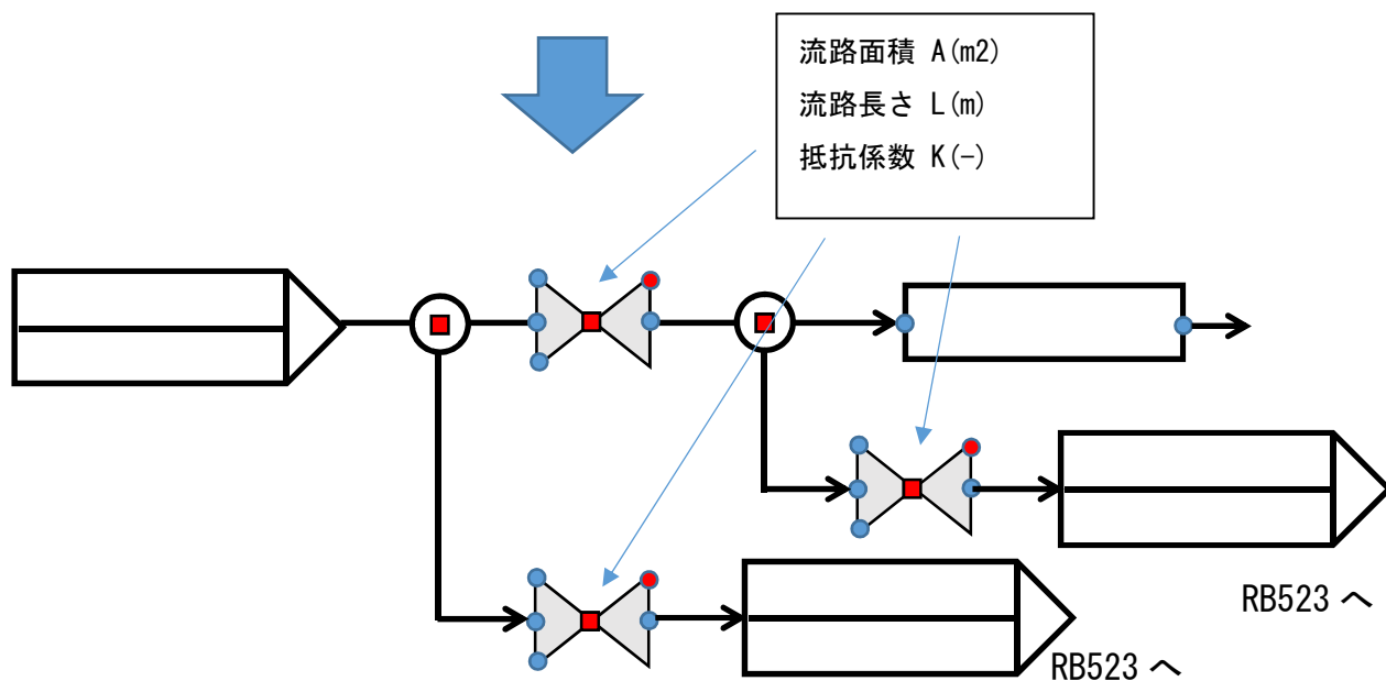
通常時 APROS モデル
