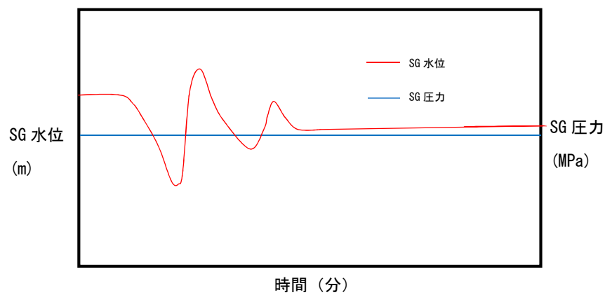
SG 水位、圧力変化図
