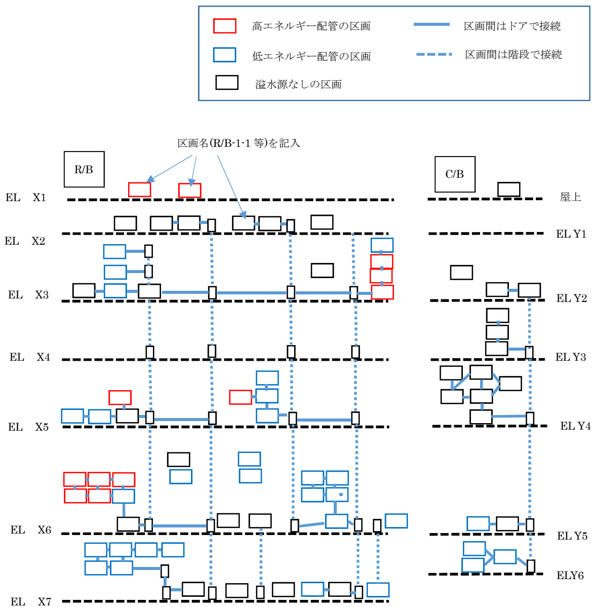
図 4.1-1 APROS モデルの作成例
