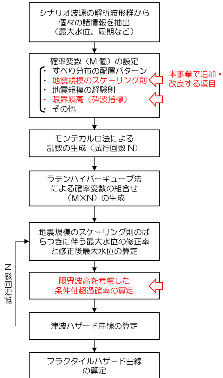
図 1 限界波高を考慮した確率論的津波ハザード解析の概略フロー
