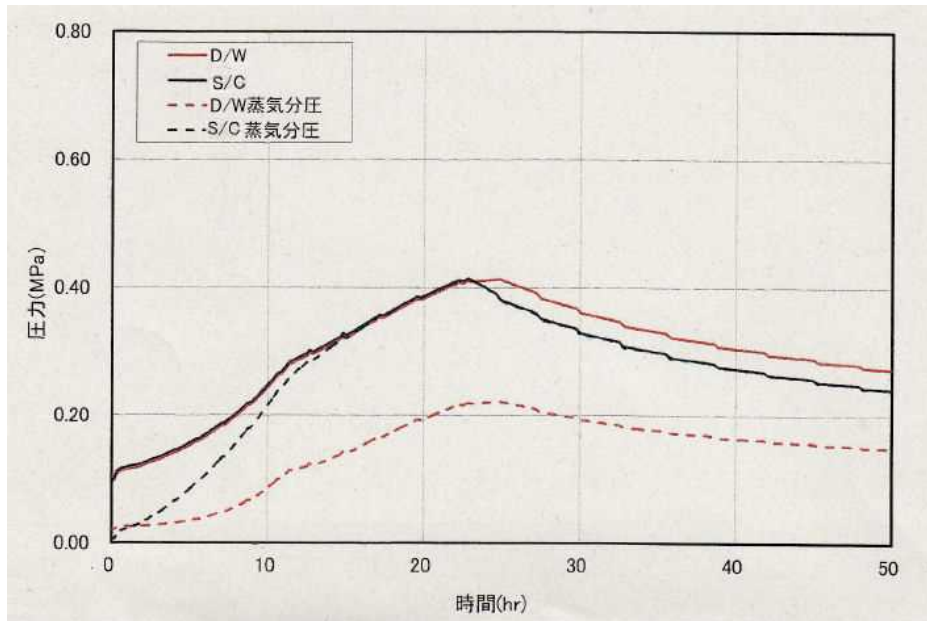
図5 TRACE5.0 コードによる格納容器挙動の解析結果の例 (D/W: ドライウェル、S/C: サプレッション・チャンバ)
