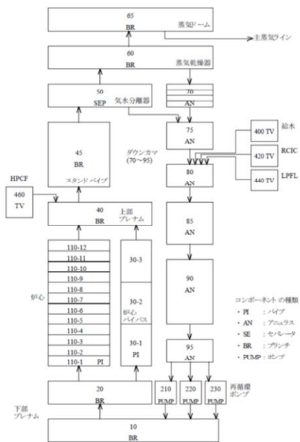
図2 RELAP5コードによるABWRプラントのモデル化の例
