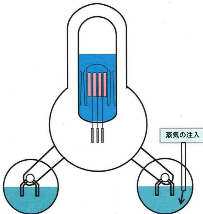
図6 サプレッション・プールへの蒸気の流入の説明図
