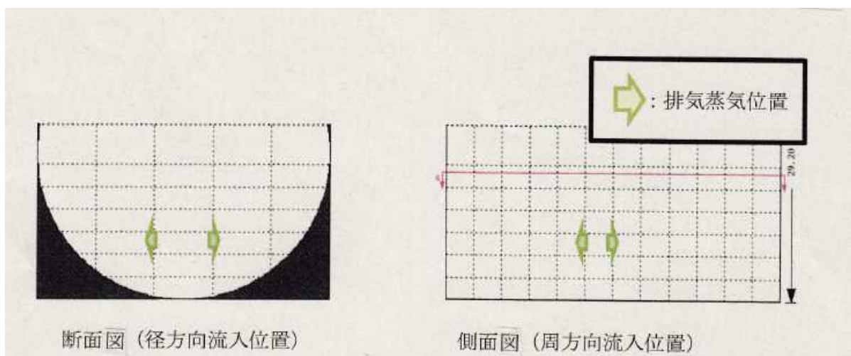
図 8 GOTHIC コードの格納容器のサブボリューム分割の例
