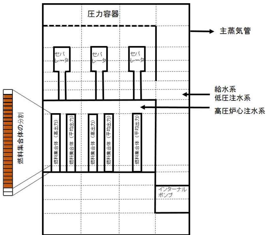
図1 TRACE5.0コードによるABWRプラントのモデル化の例
