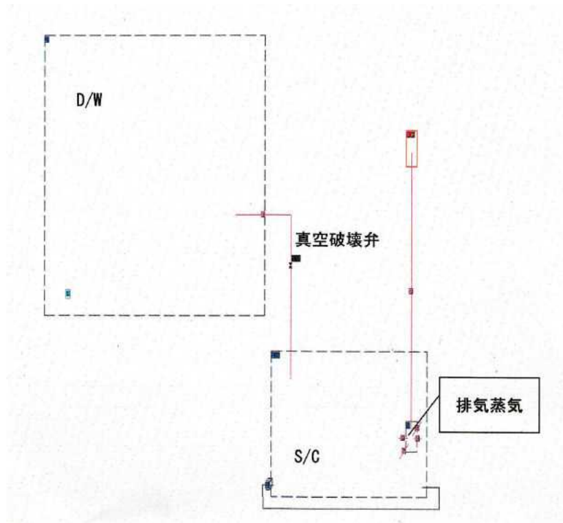
図 7 GOTHIC コードの BWR の格納容器のノード分割の例
