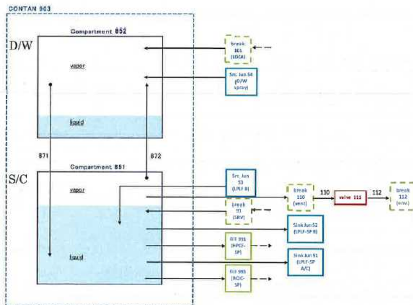
図4 CONTANコンポーネントによる格納容器のモデル化の例 (D/W: ドライウェル、S/C: サプレッション・チャンバ)
