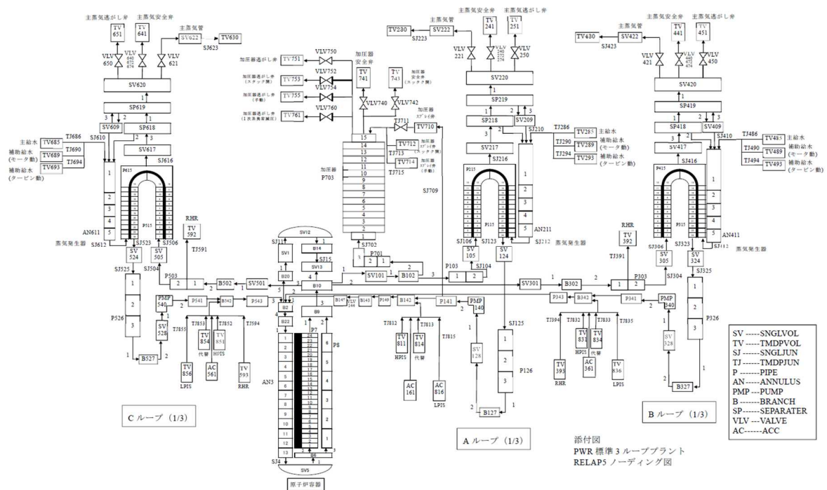
図 1 RELAP5/MOD3.3 の解析ノード分割図 (3 ループ PWR プラントデータ)
