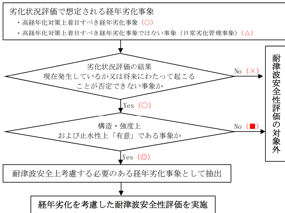
図 1 耐津波安全性評価の評価フロー
