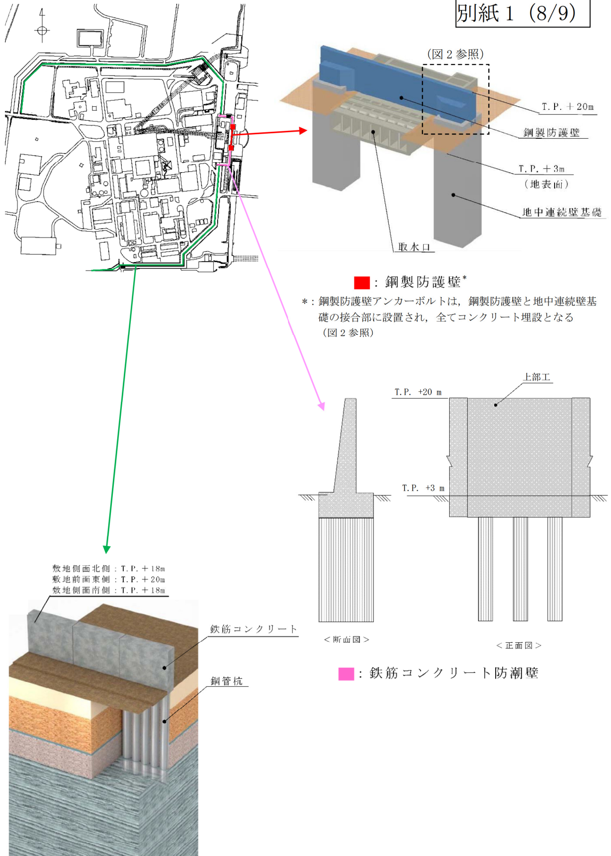
(鋼管杭鉄筋コンクリート防潮壁)
