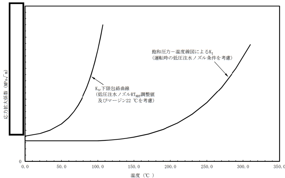
原子炉压力容器 K_{IC} 下限包絡曲線と K_I 曲線 (低圧注水ノズル: 炉心臨界時)
