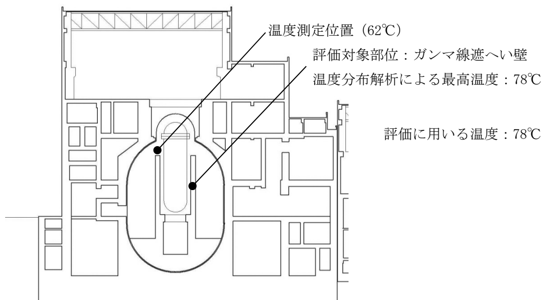
図-別紙8-2 熱によるコンクリートの遮へい能力低下 評価温度概要
