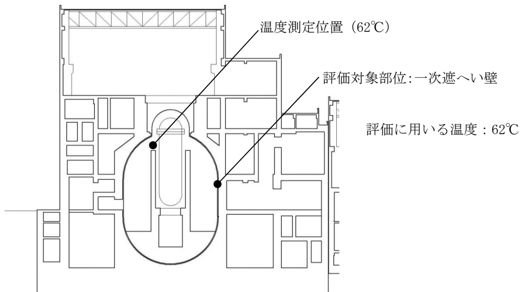
図-別紙8-1 熱によるコンクリートの強度低下 評価温度概要
