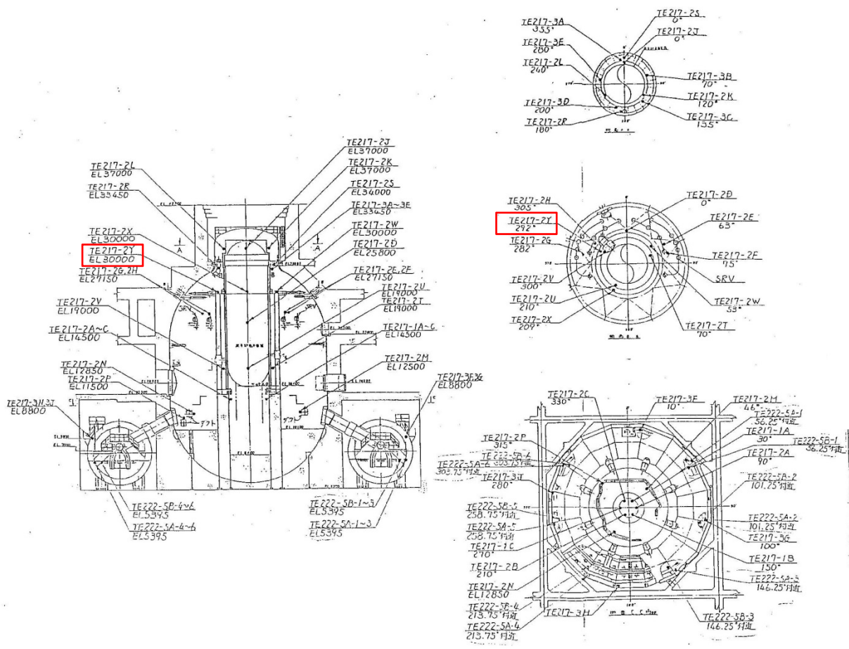
図-別紙 2-1 原子炉格納容器内雰囲気温度計検出点位置
